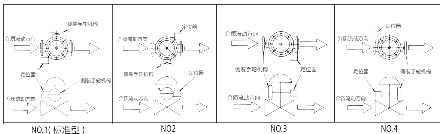
图 6 配管安装示意图
