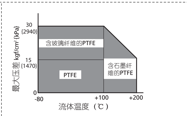
图 4. 软密封型的工作温度和最大压差范围
