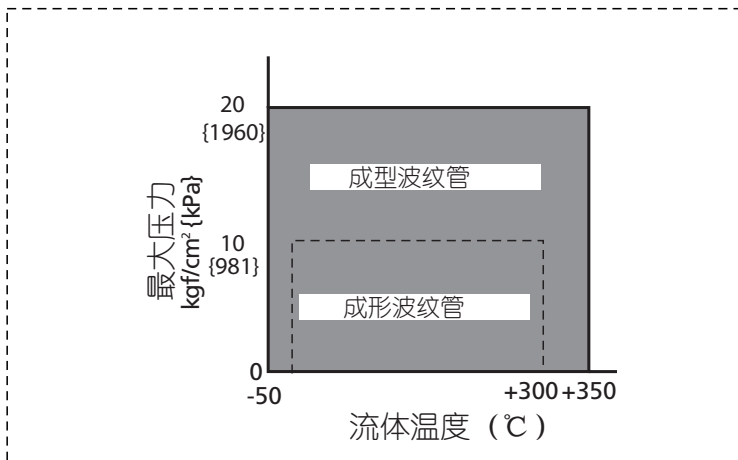
图 3 波纹管型上阀盖的工作温度和压力范围
