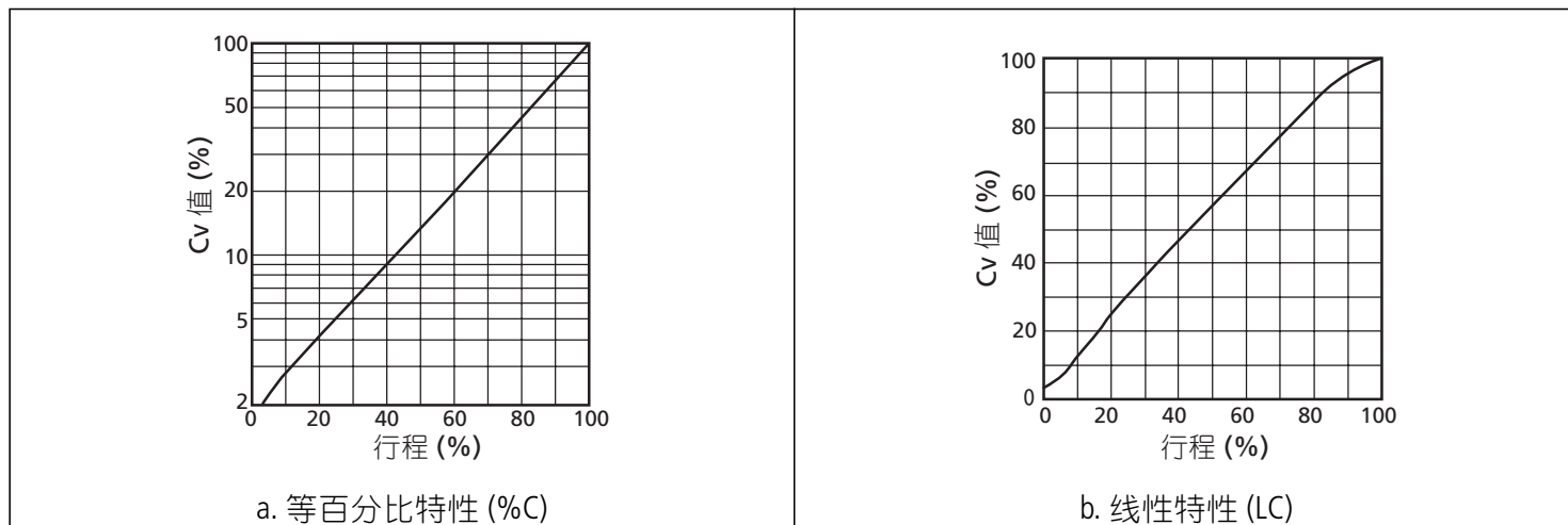
图 1 流量特性
