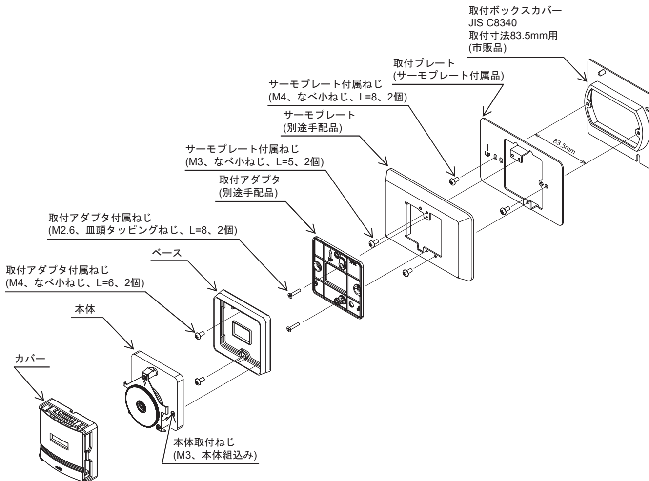
図7 サーモプレート取付
