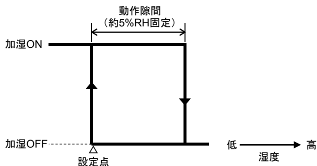
図19 形番HY6000Z2000のスイッチ動作図(加湿)
