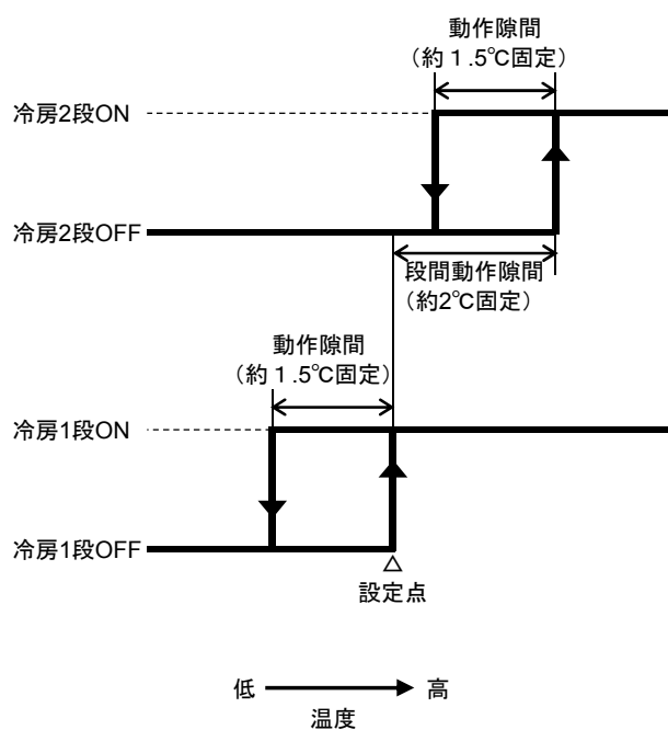
図17 形番TTY6023Z2000のスイッチ動作図(冷房)
