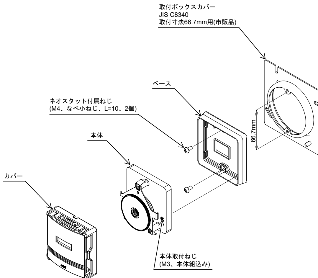
図4 壁直接取付 (新規取付の場合)
