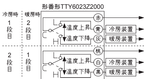
図11 結線図 形番TTY6023Z2000
