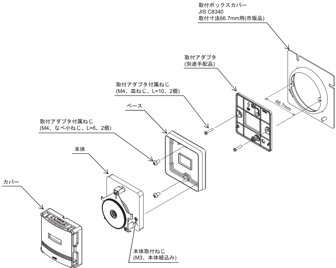
図5 壁直接取付 (既設ネオスタットからの置き換えの場合)
