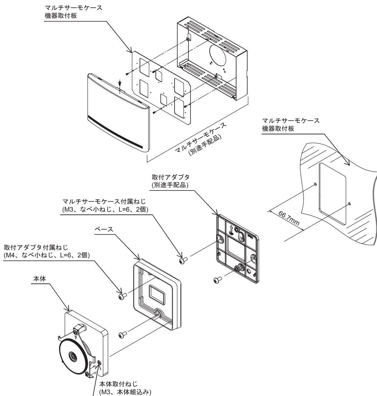
図8 マルチサーモケースへの取付
