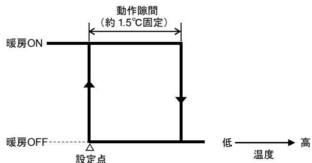
図16 形番TY600*Z2000のスイッチ動作図(暖房)
