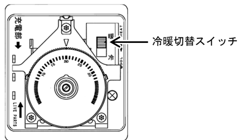
図21 冷/暖切替スイッチ (形番TY6001Z / 形番TY9001Z)
