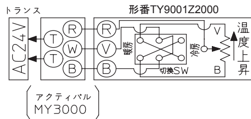
図13 結線図 形番TY9001Z2000
