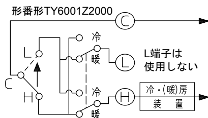
図10 結線図 形番TY6001Z2000
