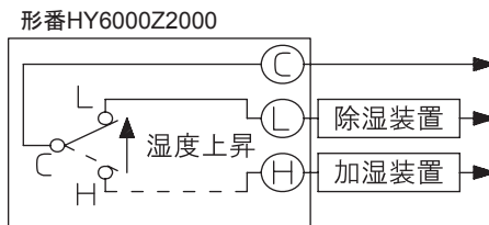
図14 結線図 形番HY6000Z2000
