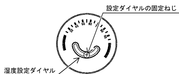
図24 湿度調節器の設定値固定
