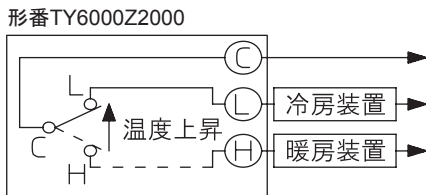
図9 結線図 形番TY6000Z2000
