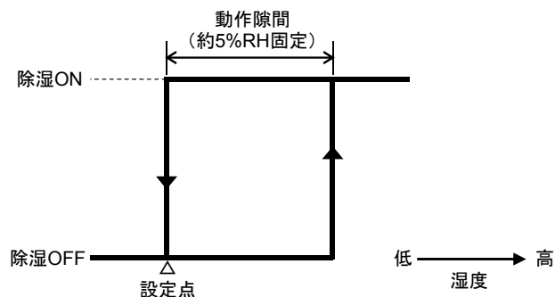
図20 形番HY6000Z2000のスイッチ動作図(除湿)
