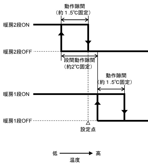
図18 形番TTY6023Z2000のスイッチ動作図(暖房)
