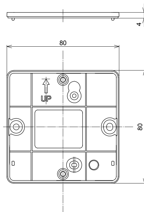
図2 取付アダプタ外形寸法 (mm)
