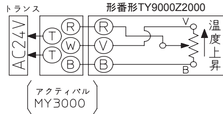
図12 結線図 形番TY9000Z2000
