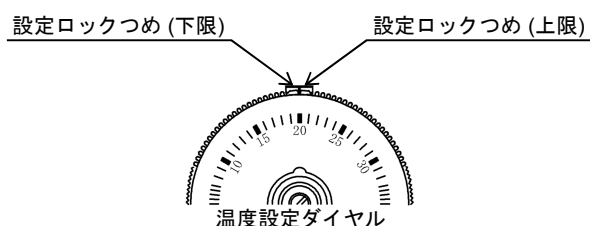
図23 温度調節器の設定値固定
