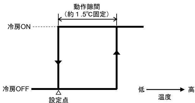
図15 形番TY600*Z2000のスイッチ動作図(冷房)
