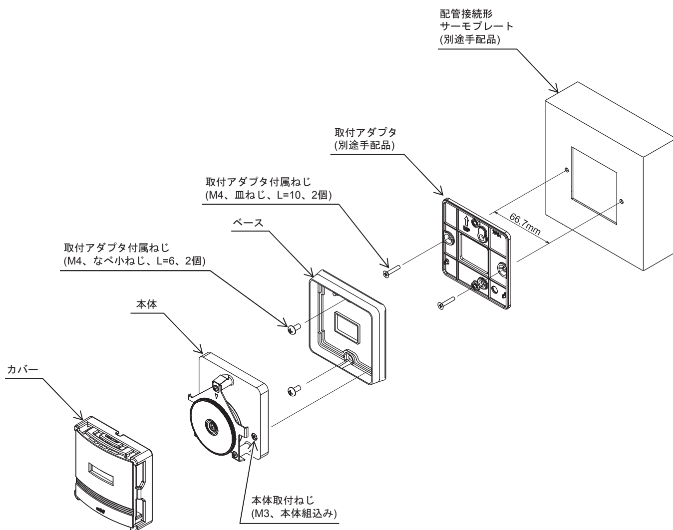
図6 配管接続形サーモプレート取付
