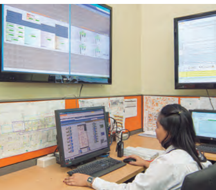
对第 1 期扩建项目天空塔区域设施进行监控的 savic-net FX 系统。有效利用太阳赌场度假酒店的网进行监控通信，除了可以减轻网络建设的负荷外，还可为今后的扩建做准备。
