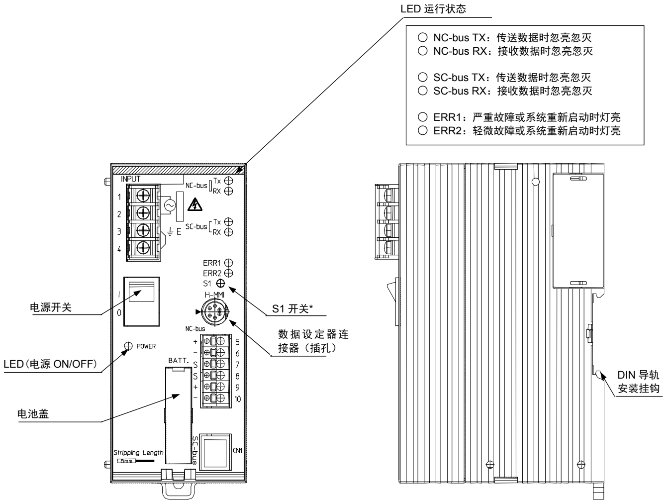
图 4 部件名称
