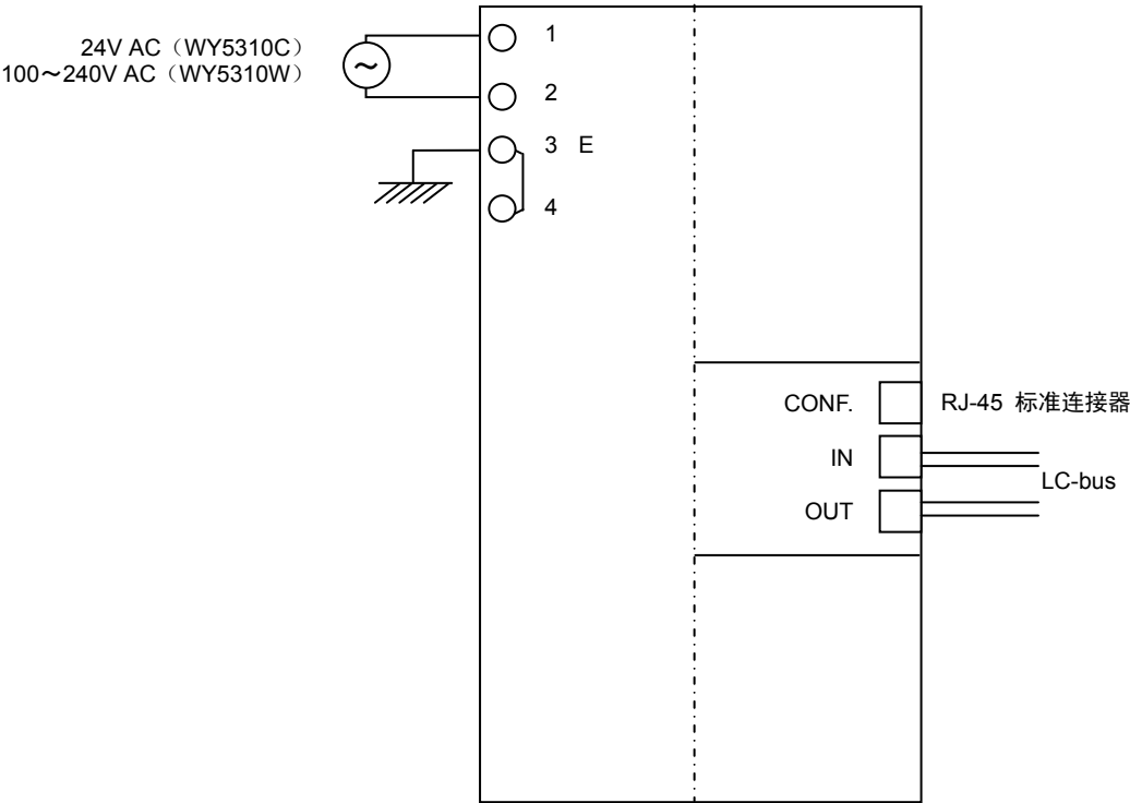
图1 输入/输出及端子配置图
