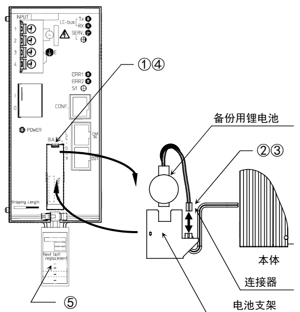
图4 电池的更换方法
