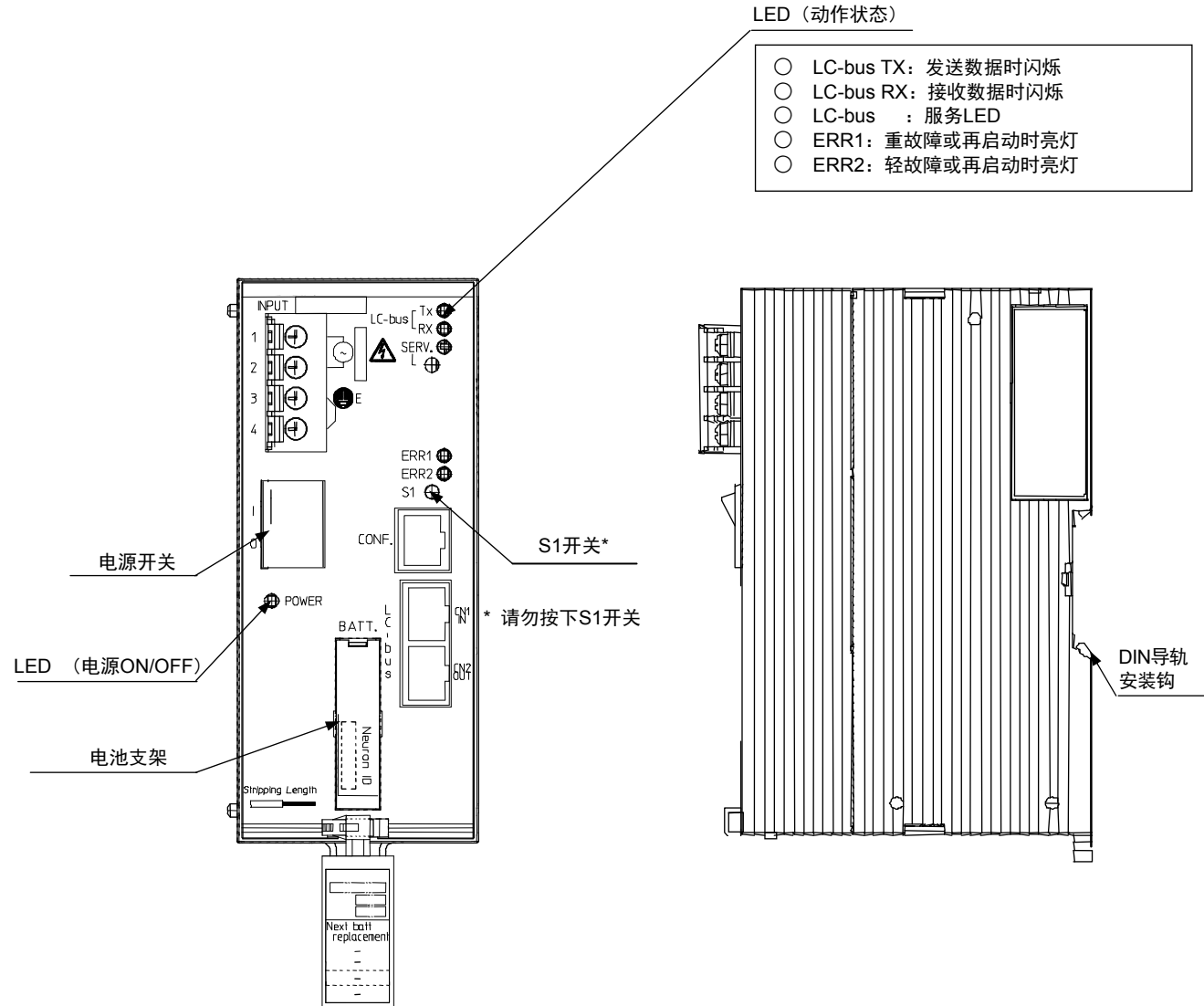
图3 各部分名称
