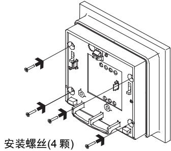
图 18. 高度变更: 固定本体
