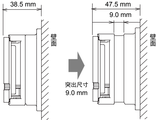
图 19. 高度变更: 本体突出的状态
