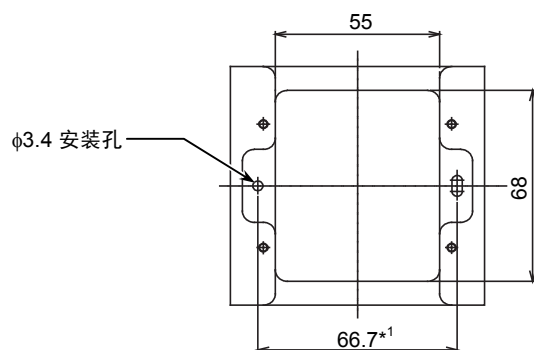
图 8. 多路隔热盒安装套件表面尺寸图 (mm)
