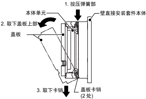
图 14. 盖板的装卸
