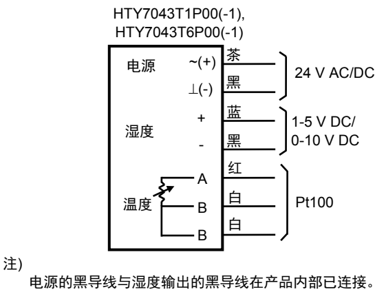
图 23. 接线图: 温湿度传感器型、Pt100、1-5V/0-10V 湿度输出、 24 V AC/DC 电源
