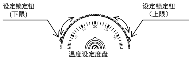
图22 温度调节器 设定值的上下限限位
