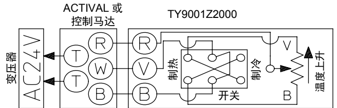
图13 接线图 TY9001Z2000
