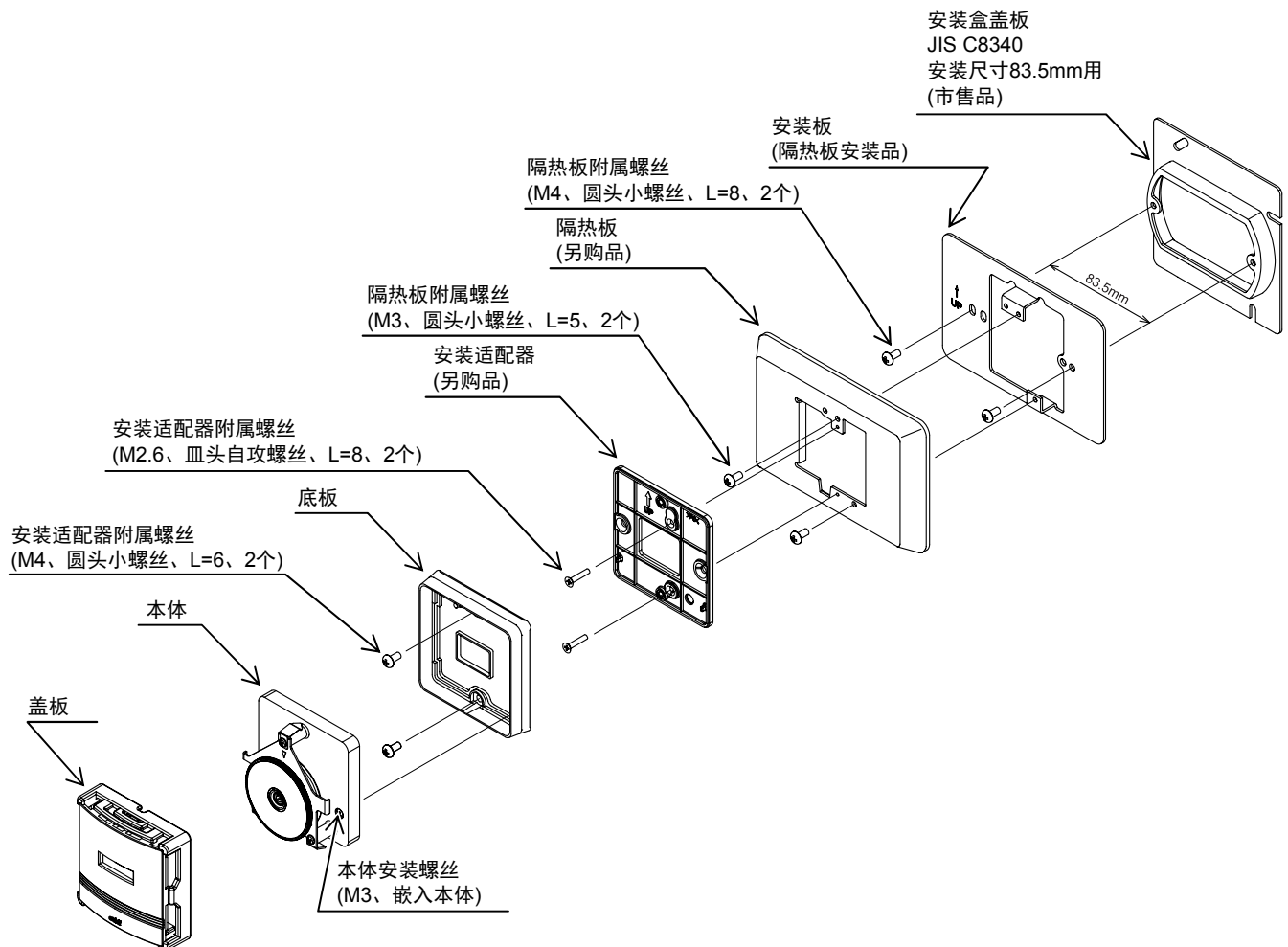
图7 安装在隔热板上
