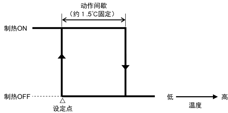
图16 TY600*Z2000的开关动作图 (制热)
