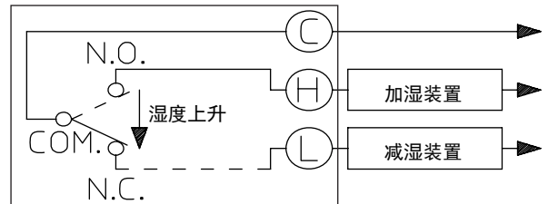
图14 接线图 HY6000Z2000
