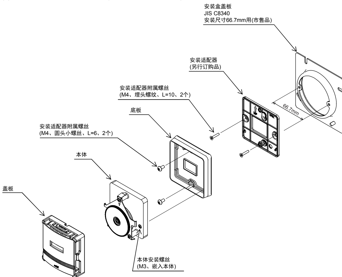
图5 壁直接安装(替换既有Neostatの場合)
