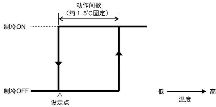
图15 TY600*Z2000的开关动作图 (制冷)
