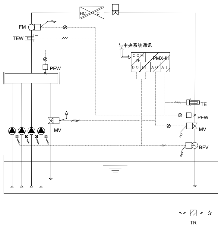
图2 开放系统自控安装实例
