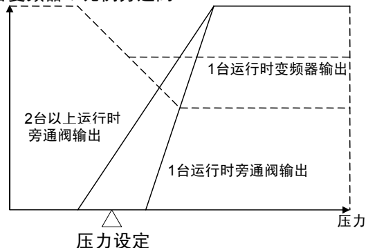
1台变频器+比例旁通阀
