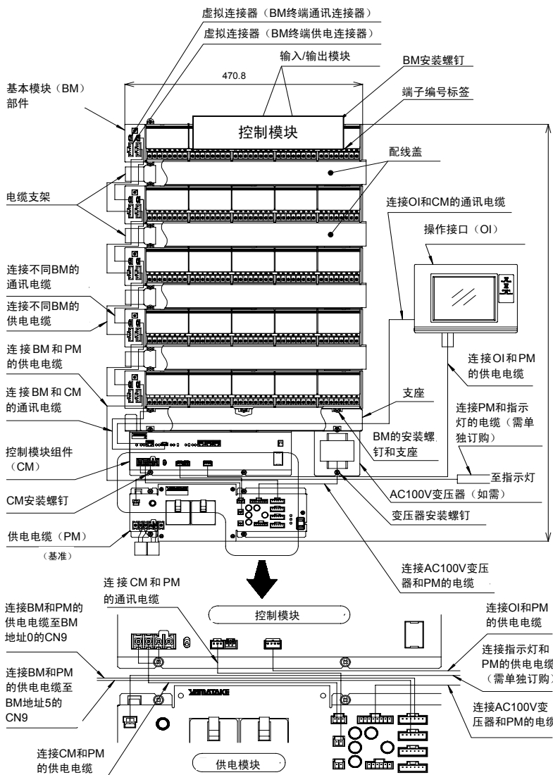
图4 设备配置图
