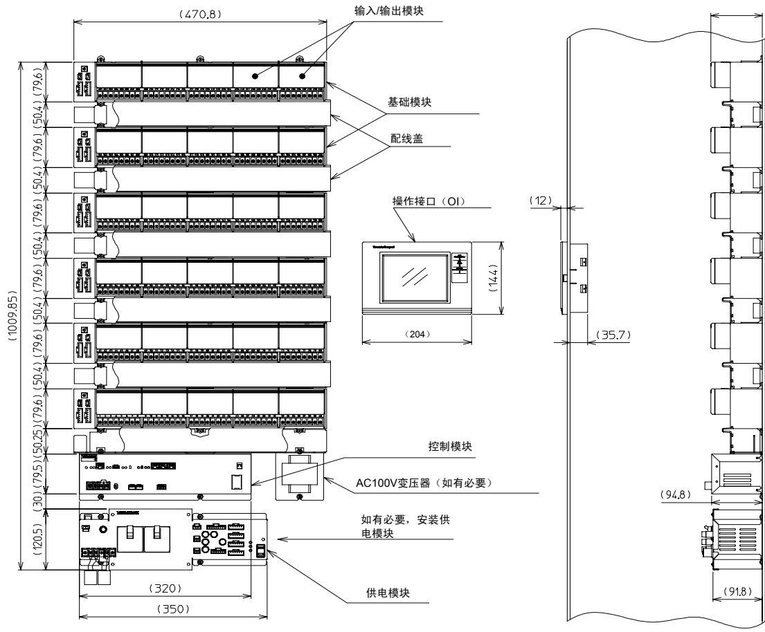
图5 外形尺寸图
