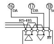
例：5 线式仪表的连接方法
