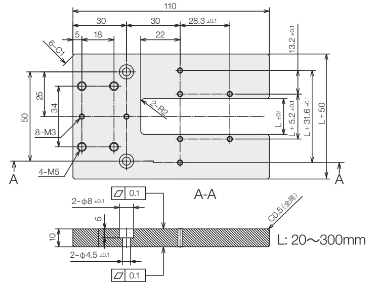
安装支架 制作参考图 型号 K1G-S07 用
