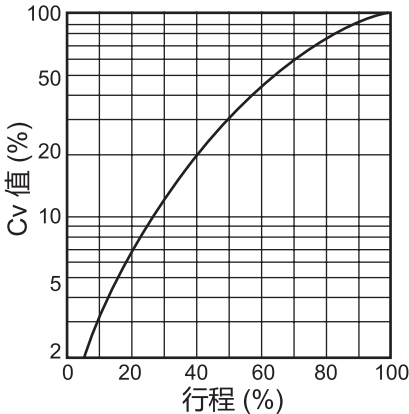
a. 等百分比特性 (%C : 金属密封, %T : 软密封)
