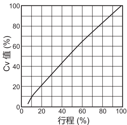
图 3-1 流量特性：高流量型 ( %CF、LCF )
