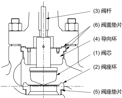
图 7-2 阀内件结构 (不带导向衬套)
