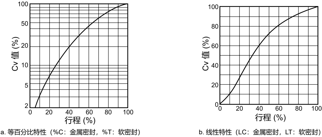
图 2 流量特性: 高容量型
