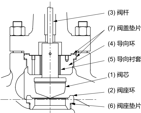
图 7-1 阀内件结构 (带导向衬套)
