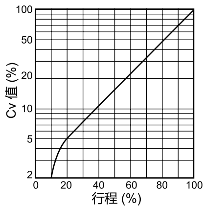
a. 等百分比特性 (%TF: 软密封)
