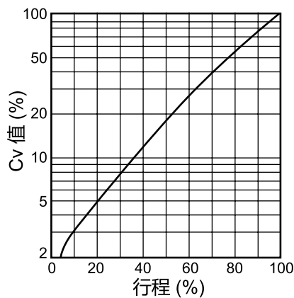
a. 等百分比特性 (%CF: 金属密封)
