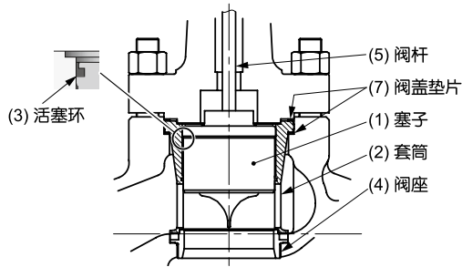
图 7-1 分体式套筒 *2
