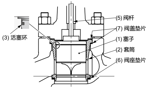
图 7-1 整体式套筒 *1
