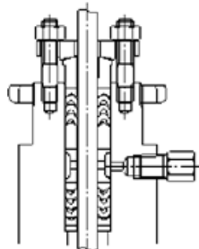
V 形 PTFE 填料 (正 + 反)
