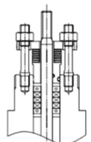
低泄漏压盖填料系统
