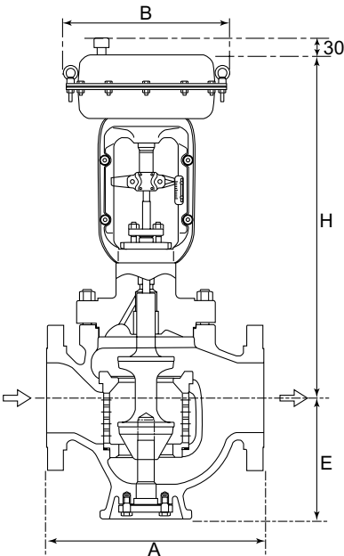
图 6 端面距和总体尺寸
