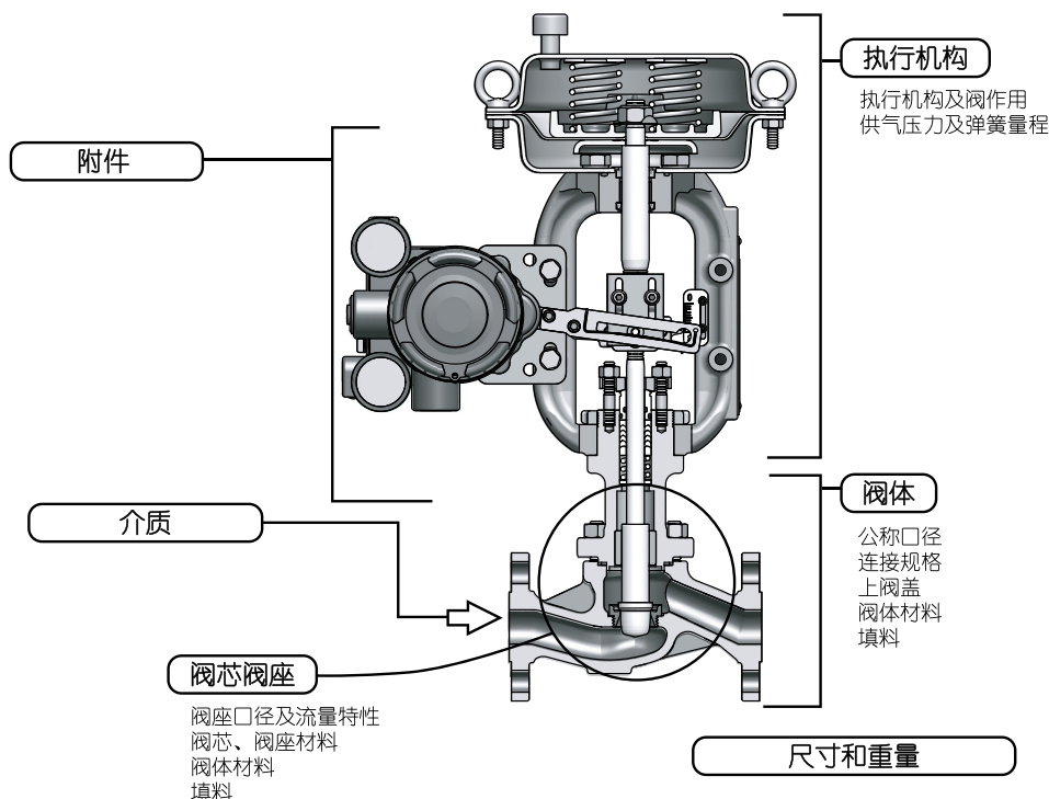
图 1 型号 AGVB/AGVM 控制阀选择项目
