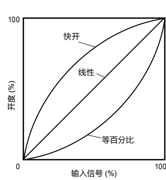
图 4. 输入/输出特性
