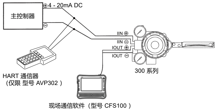
图 1. 通用电-气动定位器 (型号 AVP300/302 )
