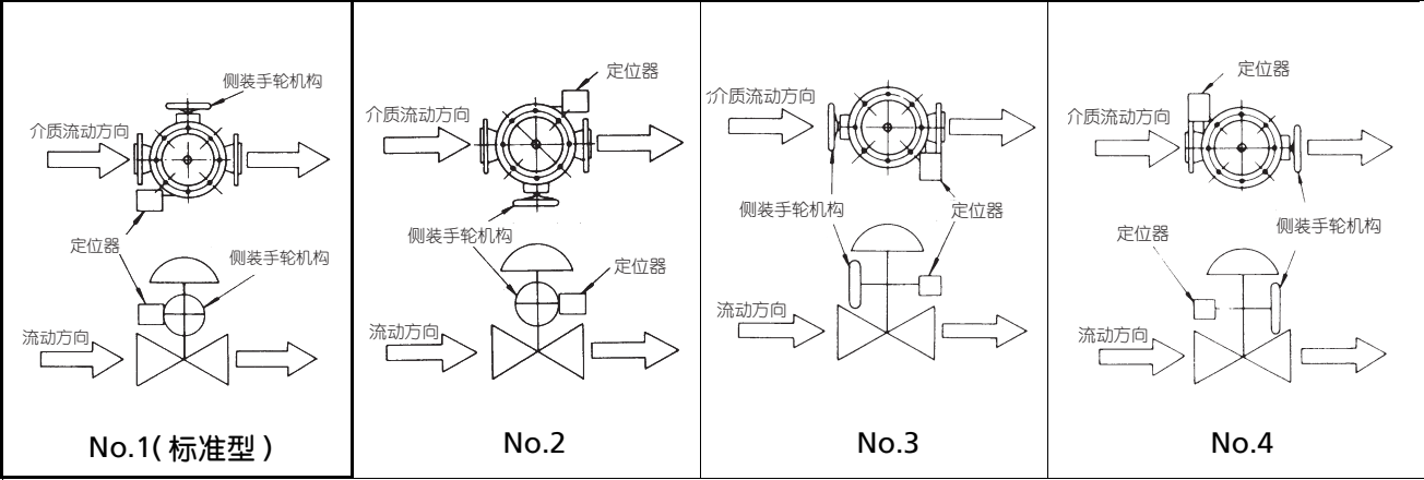
图 3 配管安装示意图
