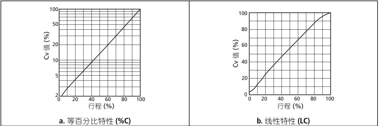
图 1 流量特性
