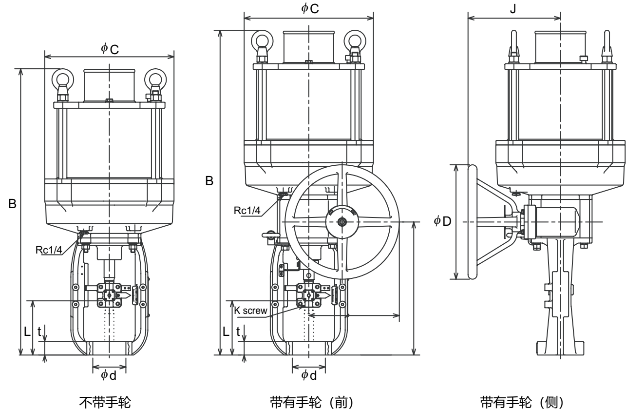
图 1 型号 PSA6R 外形尺寸
