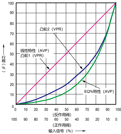
图2-2. 阀门定位器凸轮/单体的特性
