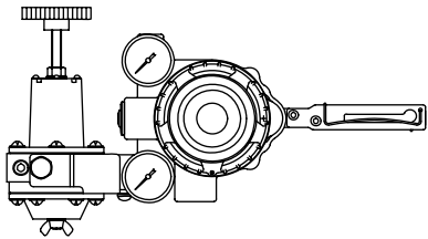
型号 AVP (一体式减压阀)
