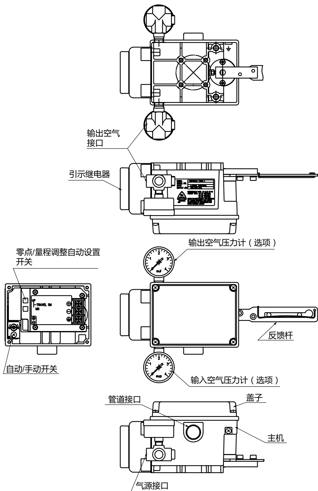
图 1-3. SVP 图
