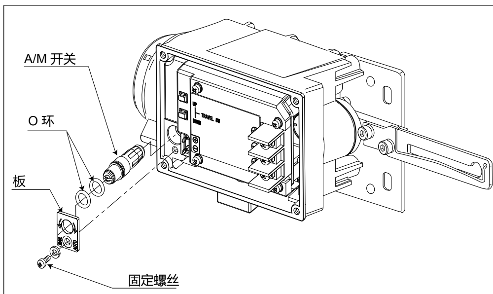
图 4-4. A/M 开关
