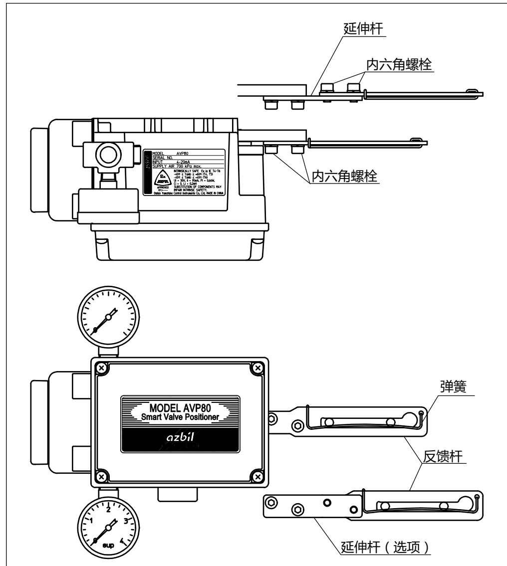
图 2-1. SVP 反馈杆
