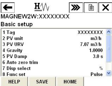
图 7-4 基本设定菜单
