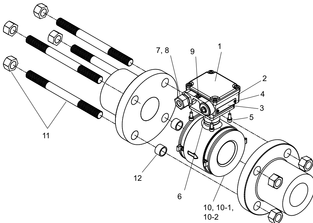
图 8-10 分离型检测器的备用零件
