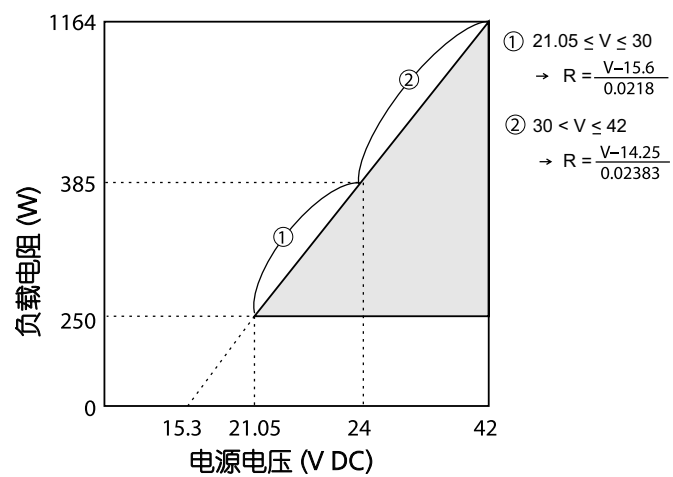
图 3-1-1 电源电压 - 负载电阻的特性
