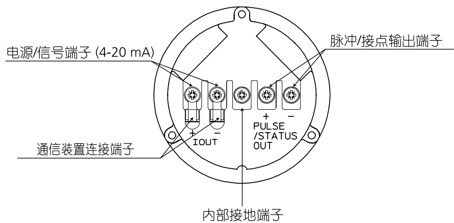
图 3-1-2 端子模块 - 一体型
