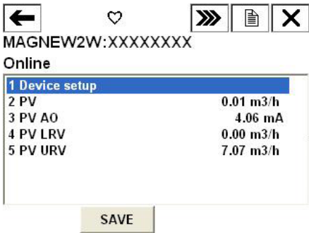
图 7-2 在线菜单
