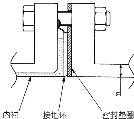
图 2-27 使用不锈钢材质接地环进行安装
