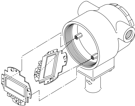
图 2-5 变更显示器 / 数据设定装置的方向
