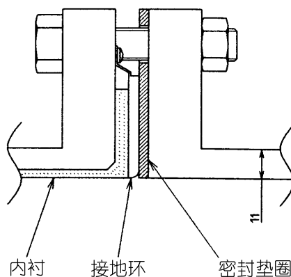
图 2-30 使用不锈钢材质接地环进行安装
