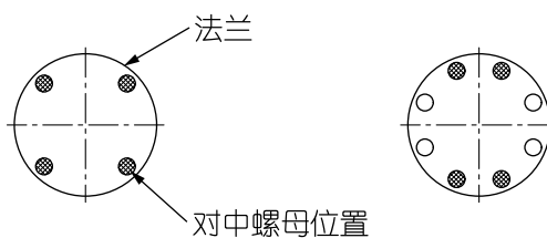
图 2-14 检测器的垂直对中 (将四个对中螺母装在底部法兰上)
