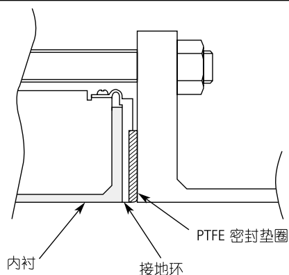
图 2-16 使用非不锈钢材质接地环和金属管道进行安装
