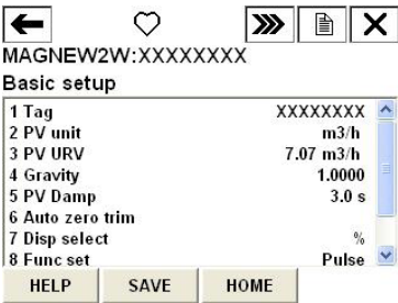
图 7-7 传输设定
