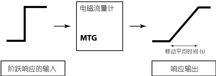
图 5-3-1 移动平均处理的输出特性
