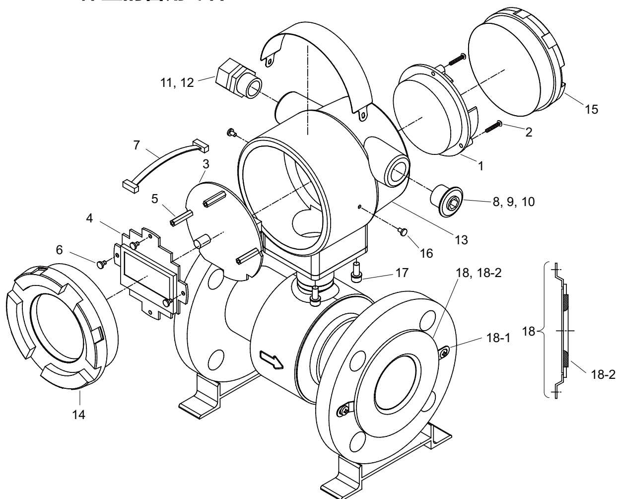
图 8-8 一体型的备用零件
