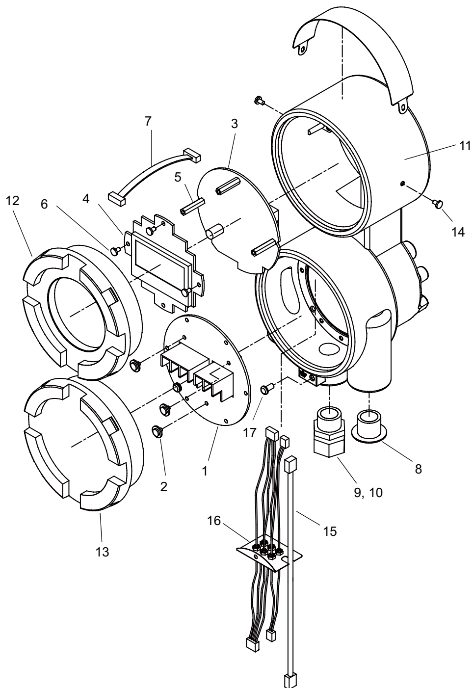
图 8-9 分离型转换器的备用零件
