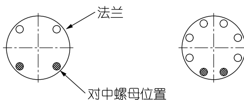
图 2-13 检测器的水平对中 (将两个对中螺母装在每个法兰上)
