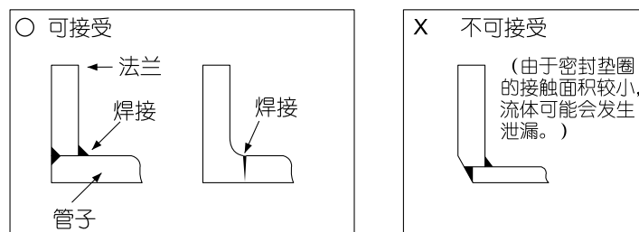
图 2-10 法兰形状
