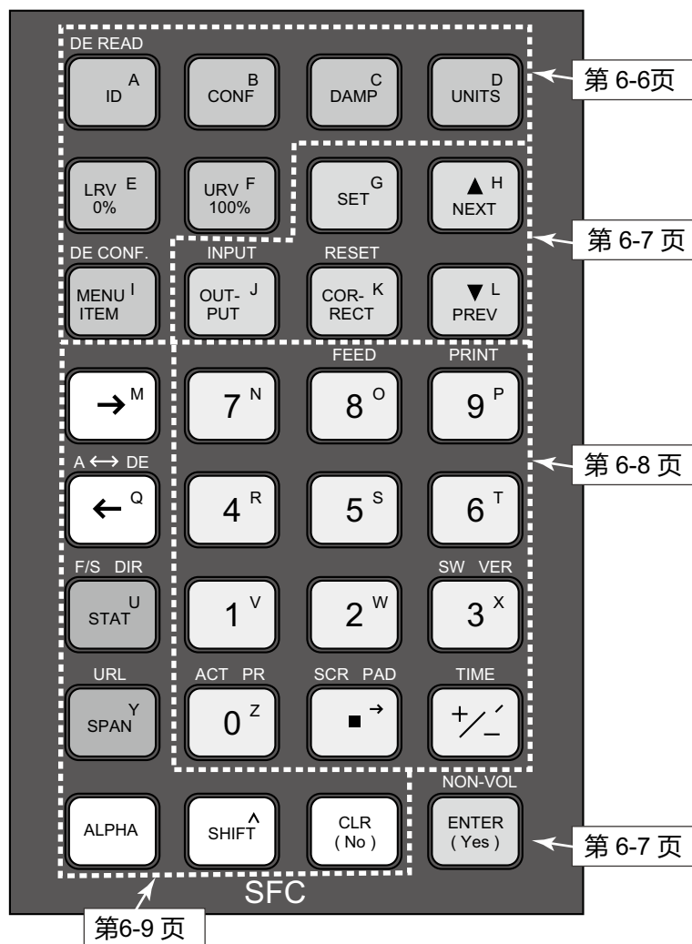
图 6-2 SFC 键盘
