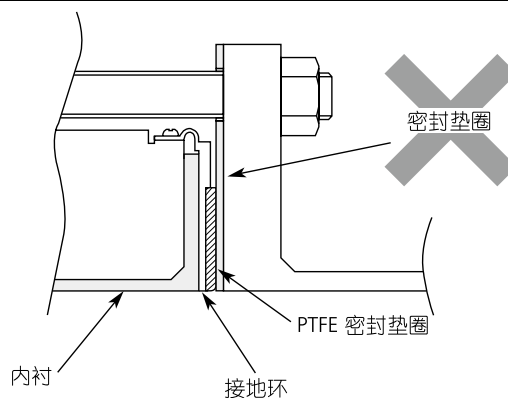
图 2-17 不正确的安装例
