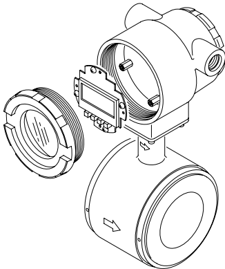
图 8-1 显示器 / 数据设定设备 (盖子已卸下) 的更换
