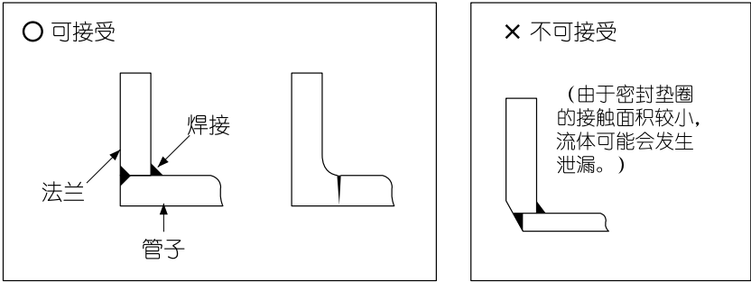
图 2-25 法兰形状
