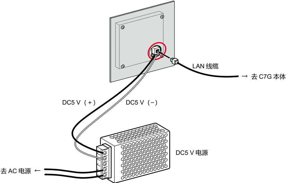
显示部端子台的配线
