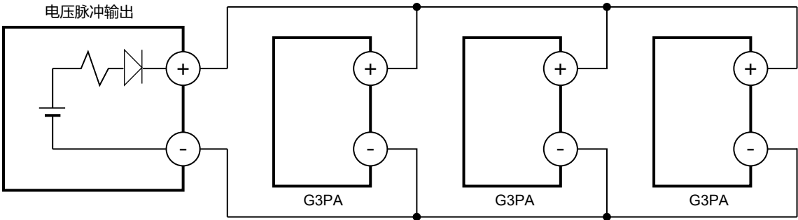
例 2：连接3台欧姆龙株式会社的G3PA的情况
