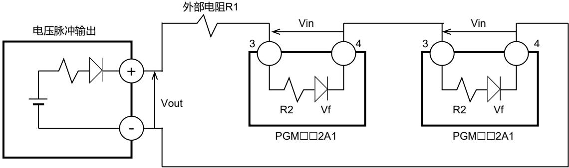
例：连接2台阿自倍尔株式会社的PGM□□2A1的情况
