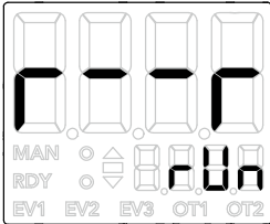
该图为参数设定 r---r 设定为 RUN/READY 切换の場合
