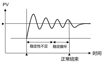
【AT时MV切换点种类=1 (SP) 的场合】
