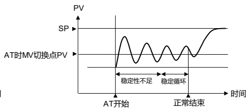
【AT时MV切换点种类=2 (PV) 的场合】
