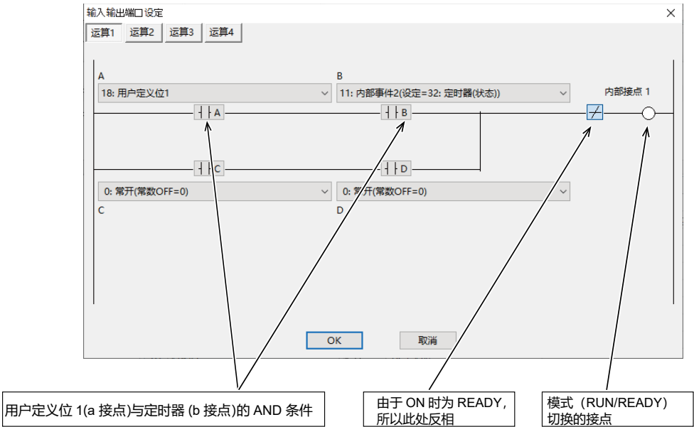
DI分配（内部接点1）：输入输出端口设定
