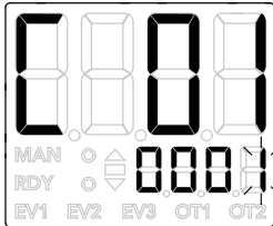
该图是 0001 的第1位正在闪烁的状态
