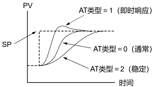
SP变更时PV变化的差异
