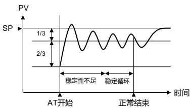
【AT时MV切换点种类=0 (默认) 的场合】
