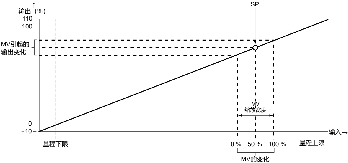
输出种类为SP + MV的场合
