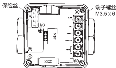
DC24V电源型
