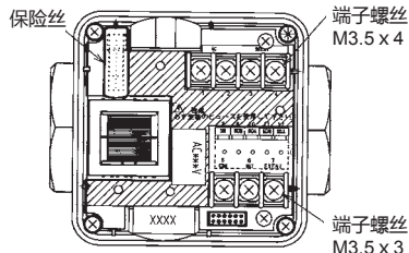
AC电源型
