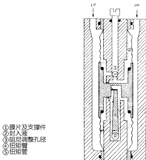
图 .6 仪表本体结构图
