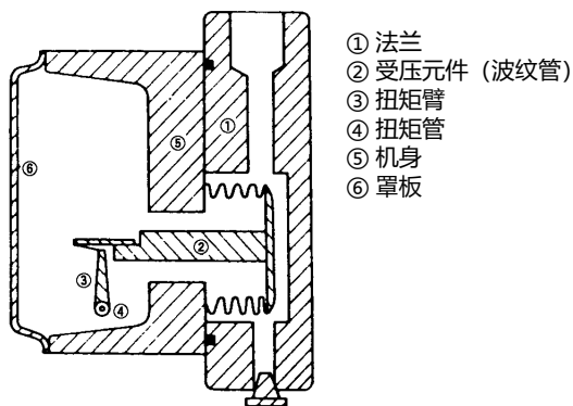
图 . 6 型号 17/18 仪表本体结构图 (波纹管元件)
