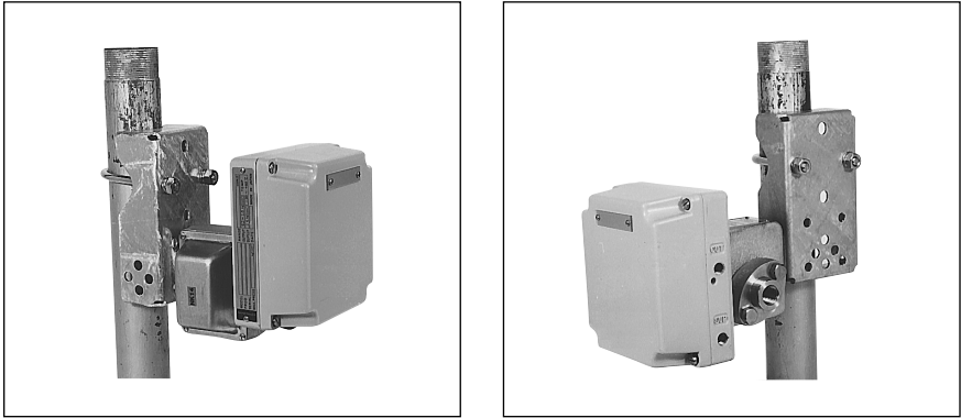
图 . 12 安装示例
