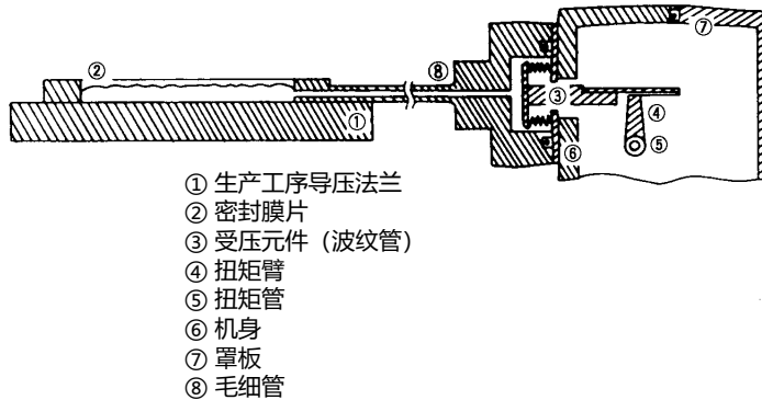
图 . 9 型号 75/76 仪表本体结构图 (波纹管元件)
