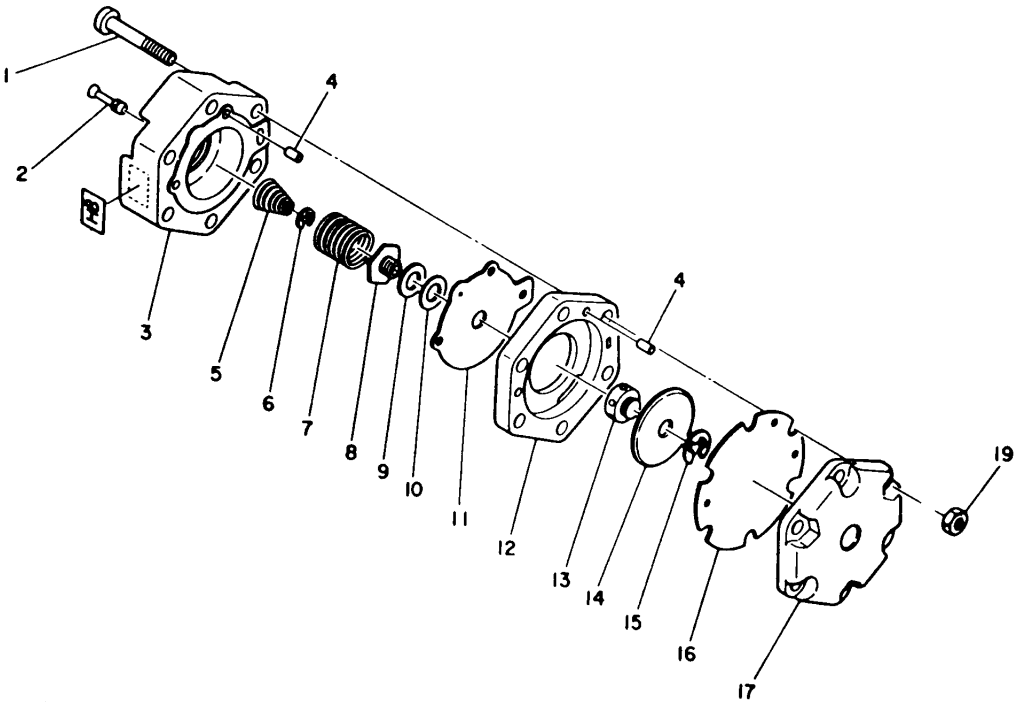
图 . 16 控制继电器分解图
