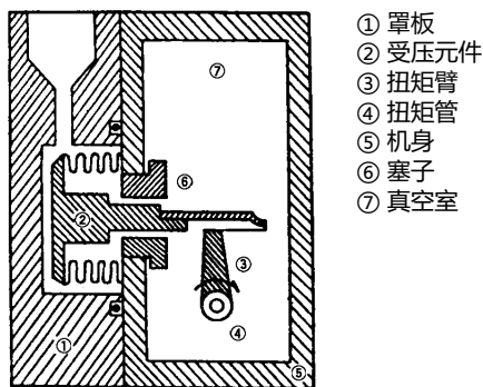
图 . 7 型号 25/26/27/28 仪表本体结构图
