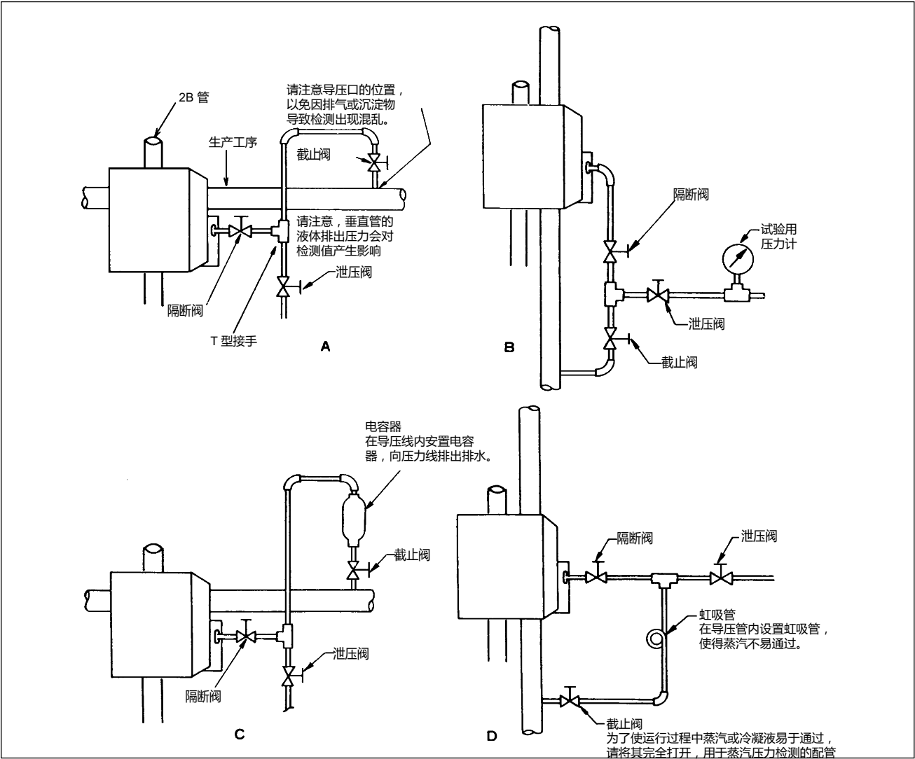
图 . 14 配管示例
