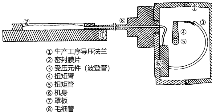
图 . 8 型号 71/72/73/74 仪表本体结构图 (波登元件)
