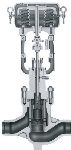
图 1-4 压力平衡高压笼式控制阀型号 HPC
