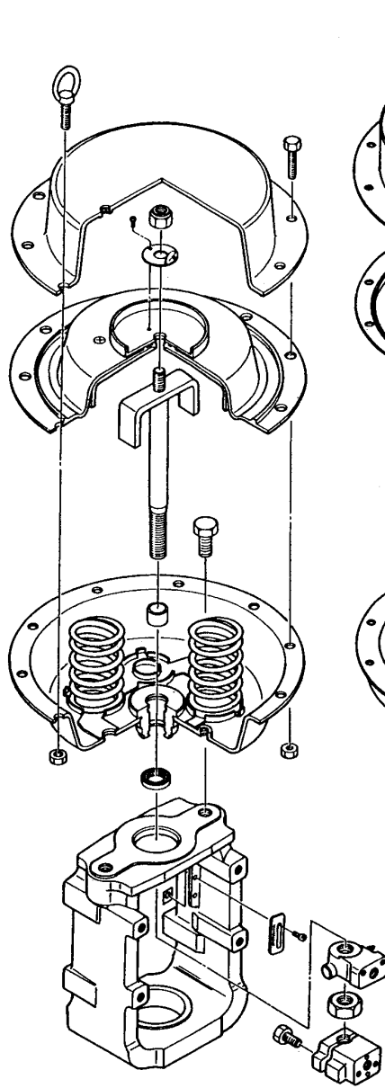
图 4-10 型号 HA2D 或 HA3D 执行机构
