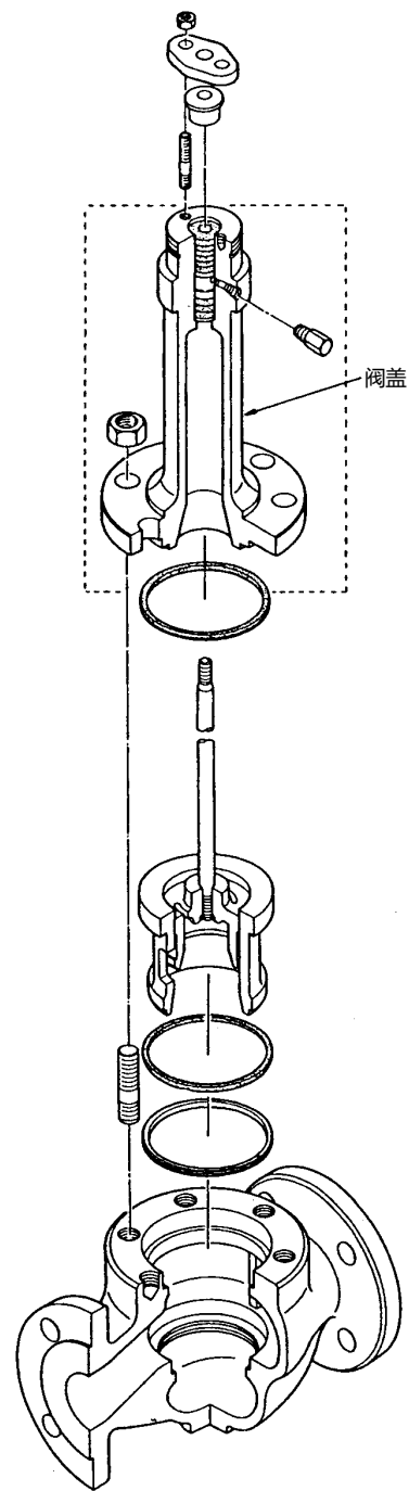
图 4-1-2 高温型 (阀盖加长型)
