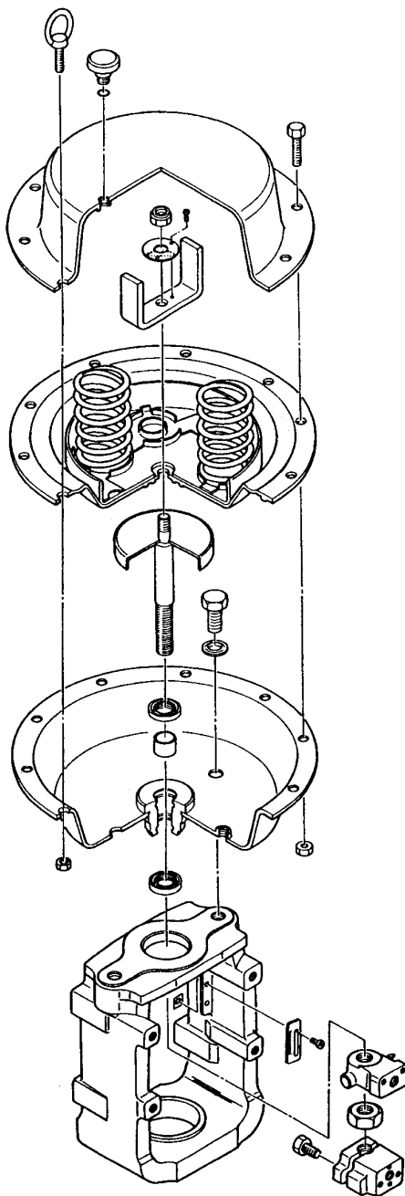
图 4-12 型号 HA2R 或 HA3R 执行机构
