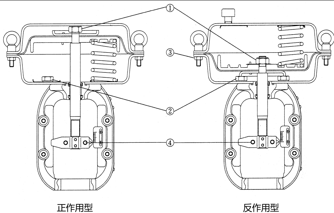
图 4-8 执行机构的螺栓和螺母
