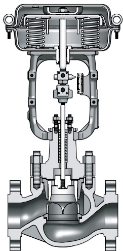
图 1-1 压力平衡笼式控制阀型号 HCB
