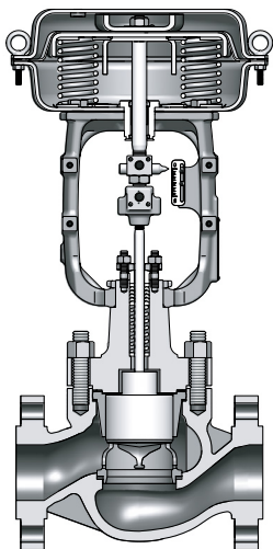
图 1-3 低噪音笼式控制阀型号 HCN
