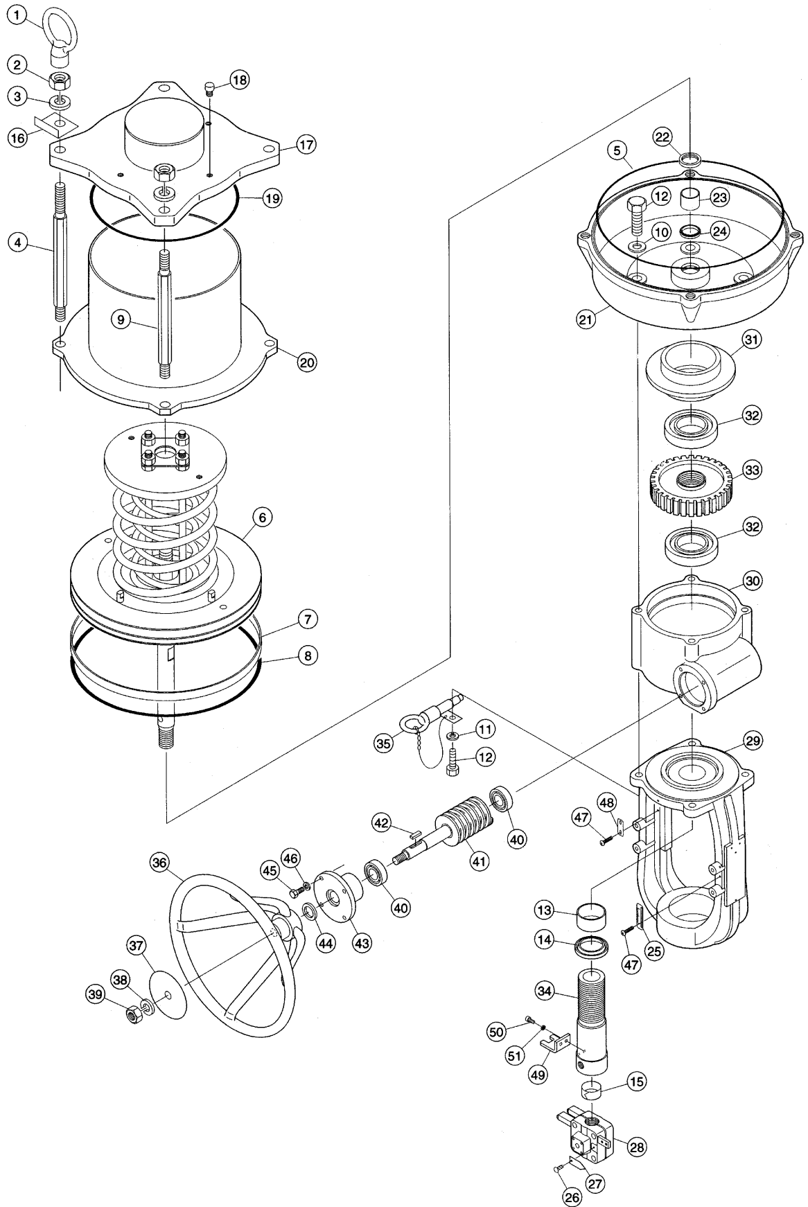
图 4-22 型号 PSA6R
