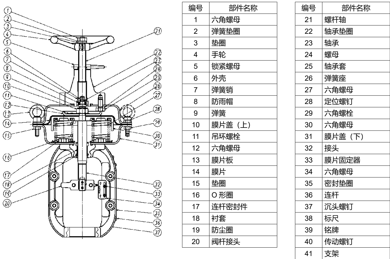
图 7-2 带顶部手轮的型号 PSA1 执行机构（反作用型）
