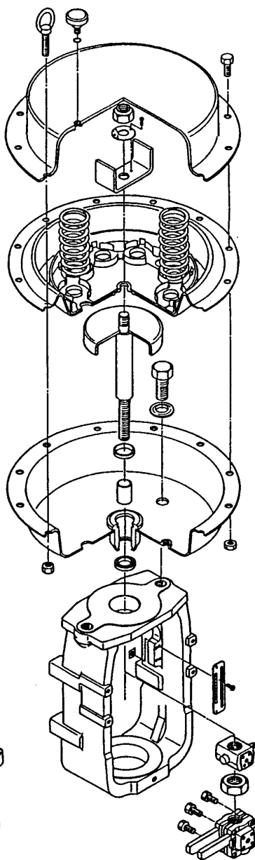
图 4-13 型号 HA4R 执行机构
