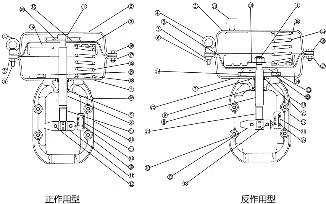
图 4-9 型号 PSA 执行机构
