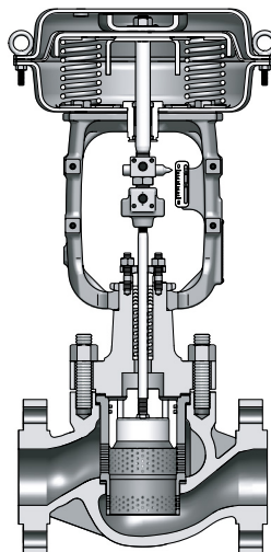
图 1-2 压力不平衡笼式控制阀型号 HCU
