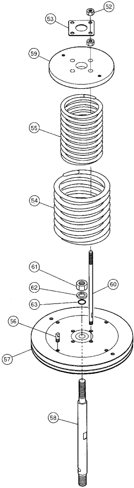
图 4-23 弹簧单元
