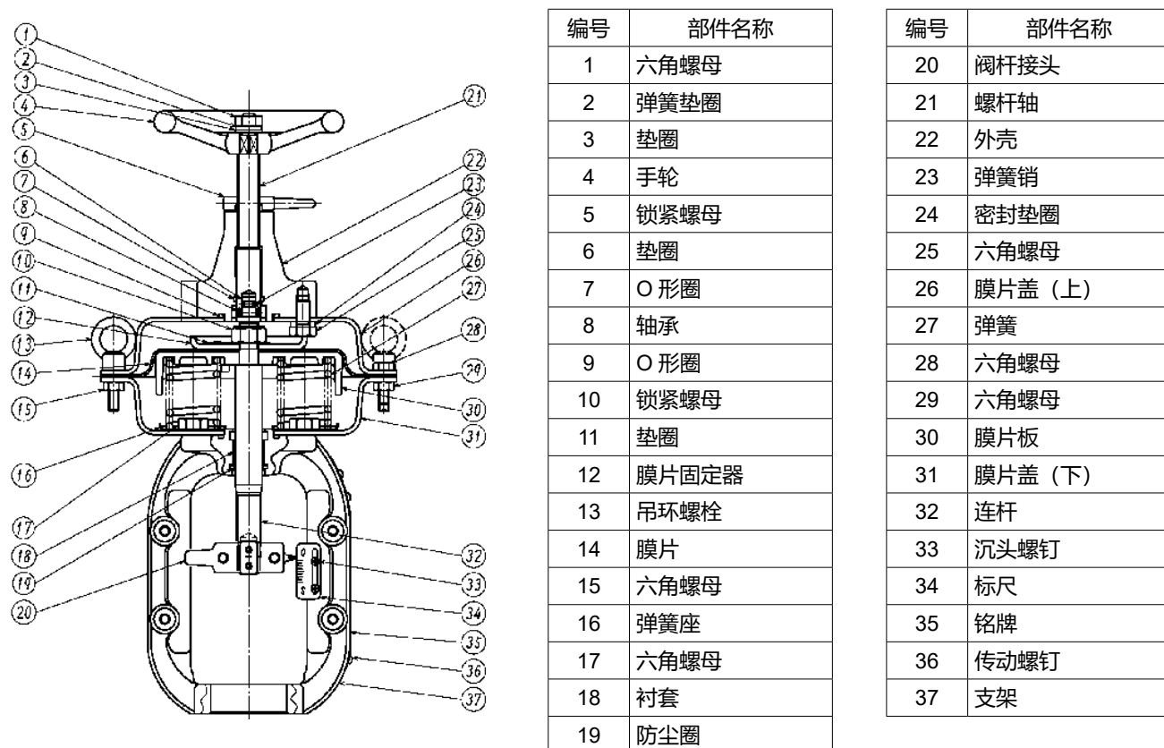
图 7-1 带顶部手轮的型号 PSA1 执行机构（正作用型）
