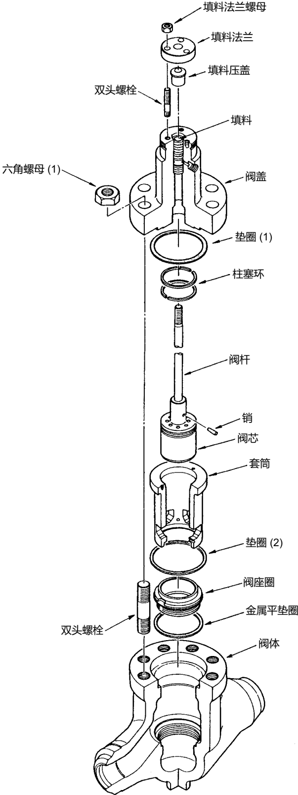
图 4-2 型号 HPC 控制阀
