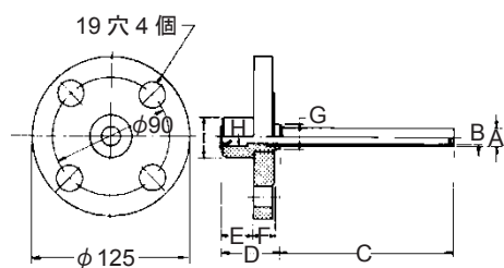
図2 外形寸法図 (形番189020B-J)
