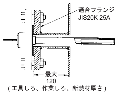
図3 フランジ形保護管取付例
