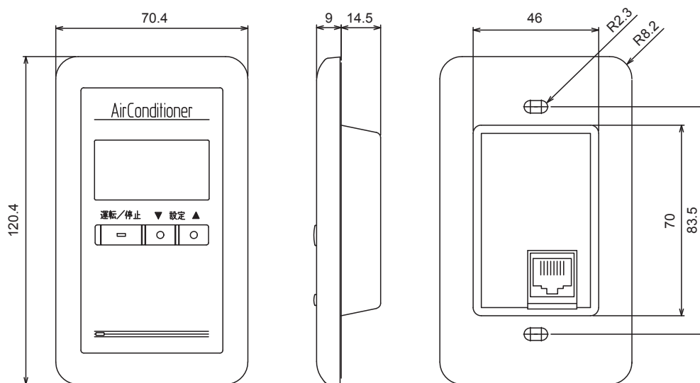
図3 ネオパネル(縦形)外形寸法図 (単位 : mm)
