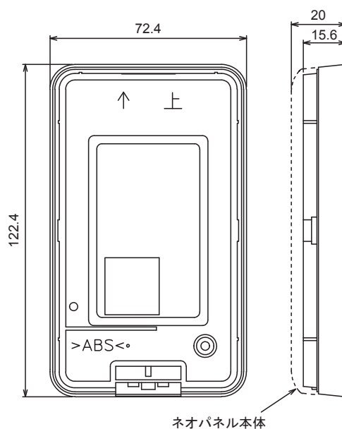
図4 サーモプレート (単位 : mm)
