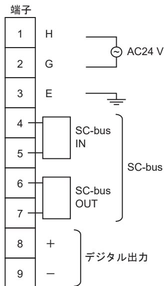
図6 結線
