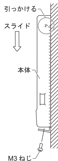
図5 ネオターミナルの取付
