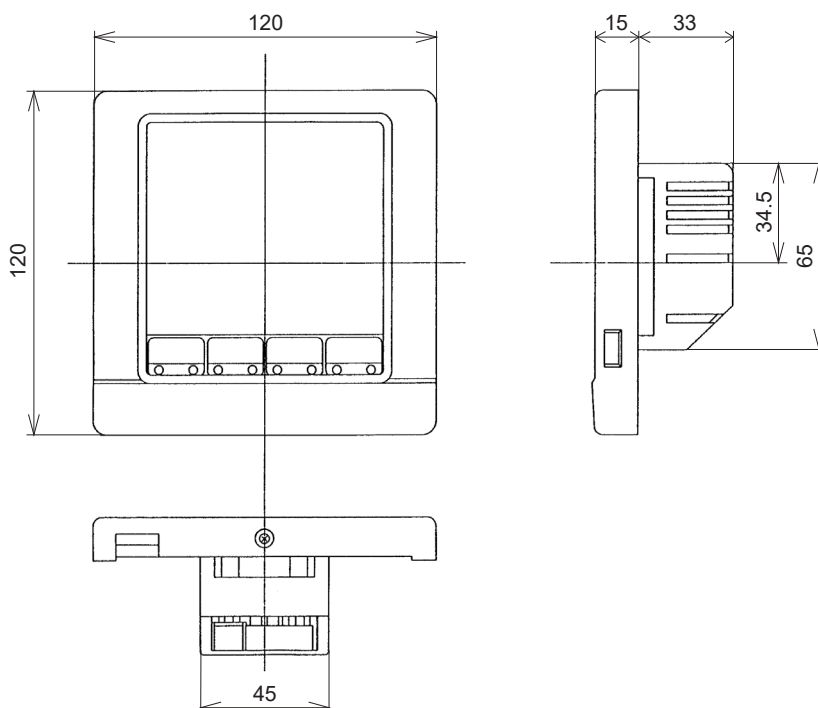
図3 外形寸法図 (mm)
