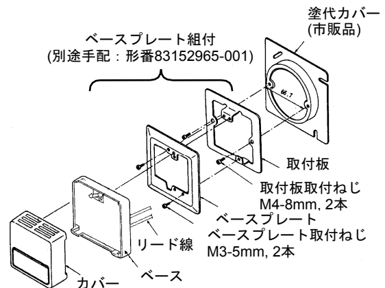
図4 取付図
