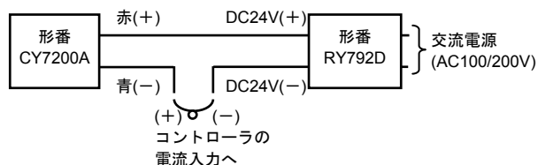
図7 結線図
