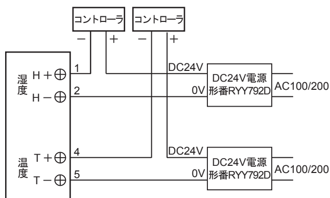
図17 形番HTY78*3D***/TY78*3D***/HY78*3D***の結線例
