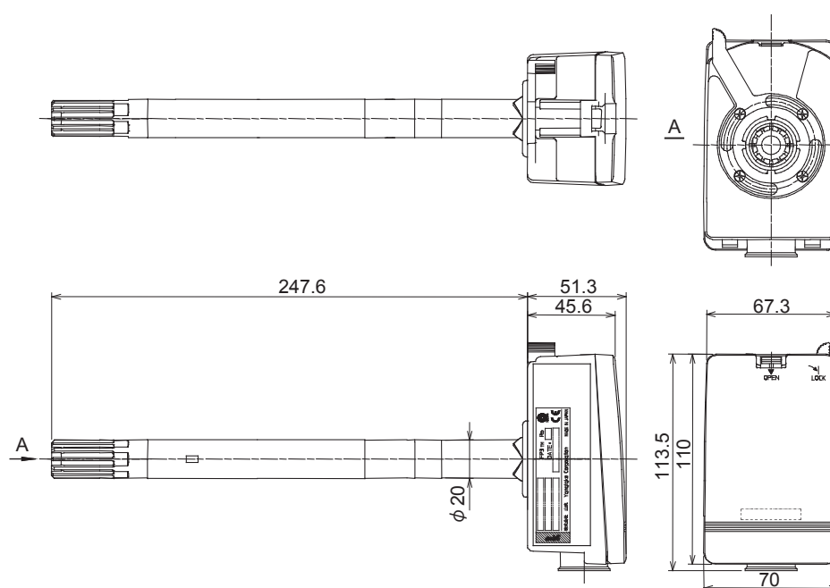
図1 挿入部：長 (形番HTY7803、形番TY7803、形番HY7803) 外形寸法図 (mm)
