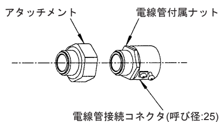
図26 電線管接続コネクタ
