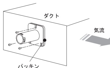
図5 ブラケットの取付
