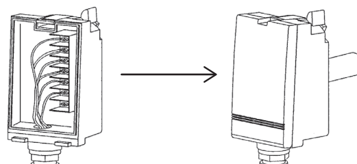
図28 カバーの取付
