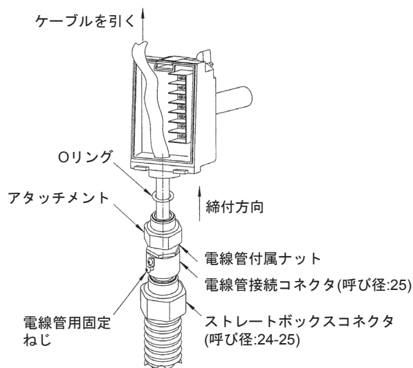
図27 電線管接続
