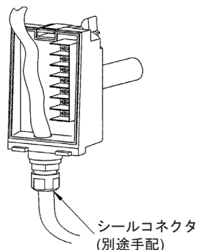
図25 シールコネクタ接続
