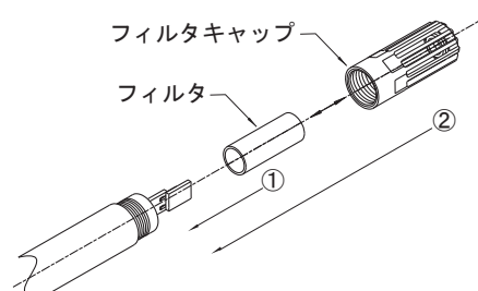
図33 フィルタの取り付け
