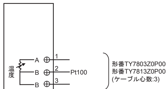
図15 端子番号とケーブル心数 (形番TY78*3Z0P00)
