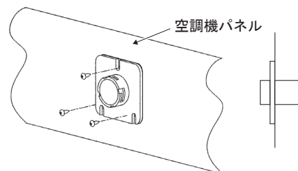
図10 ブラケットの取付
