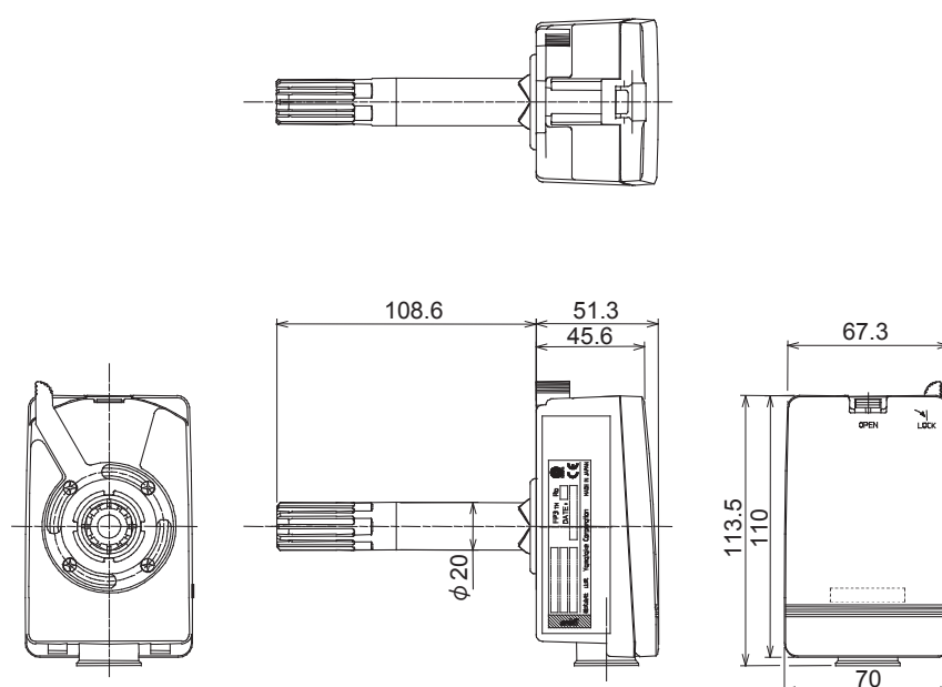
図2 挿入部：短 (形番HTY7813、形番TY7813、形番HY7813) 外形寸法図 (mm)
