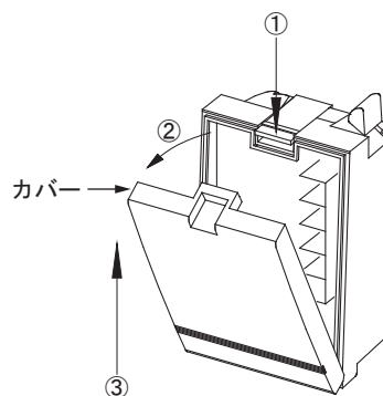
図24 カバーの取外し
