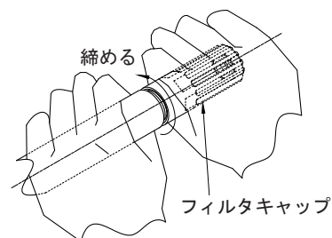
図34 フィルタキャップの取り付け
