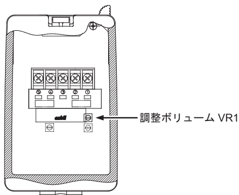
図36 調整ボリュームの位置 (形番HTY/HY78*3D)
