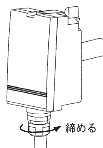
図29 シールコネクタ
