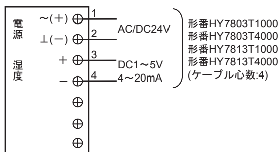
図14 端子番号とケーブル心数 (形番HY78*3T*000)
