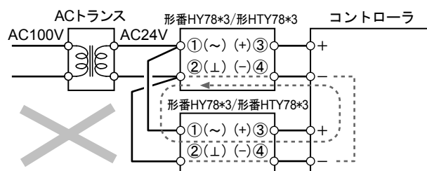
図22 回路内にループができた場合
