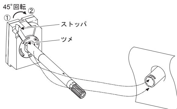
図7 本体の取付
