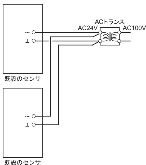
図20 置き換え前の配線
