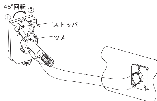
図11 本体の取付
