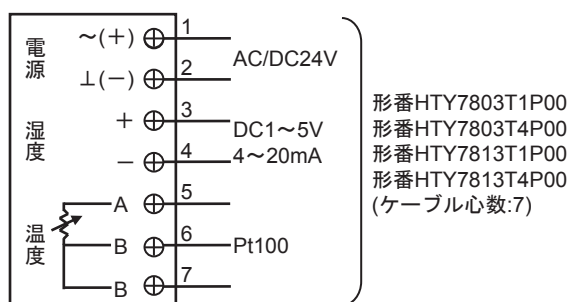
図13 端子番号とケーブル心数 (形番HTY78*3T*P00)
