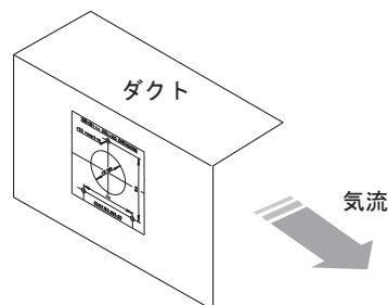
図4 穴あけ
