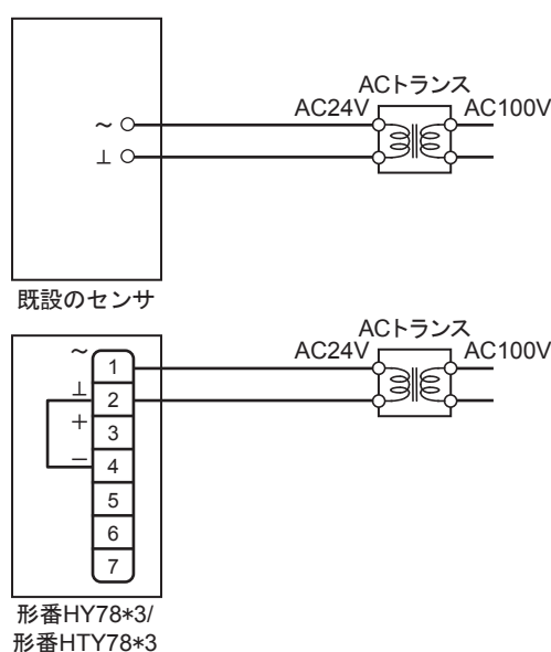
図21 置き換え後の配線
