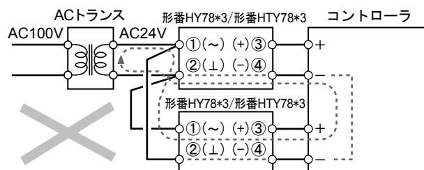
図23 誤配線した場合
