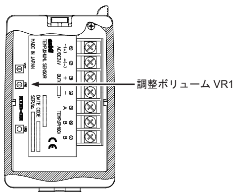
図35 調整ボリュームの位置 (形番HTY/HY78*3T)
