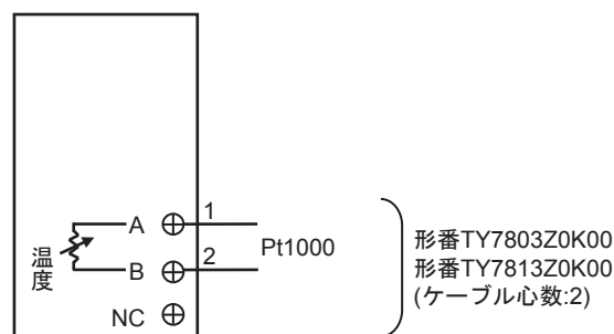
図16 端子番号とケーブル心数 (形番TY78*3Z0K00)
