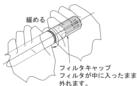
図30 フィルタの取り外し
