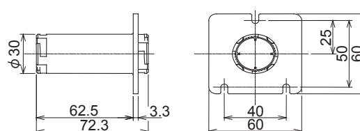
図3 取付ブラケット (mm)
