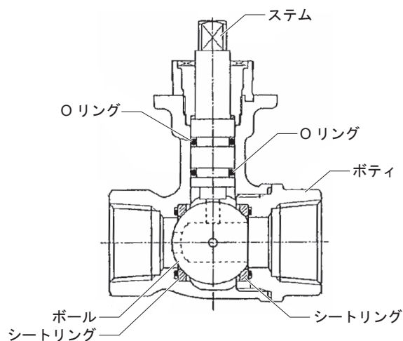
図2 各部の名称
