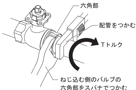
図6 配管への取り付け
