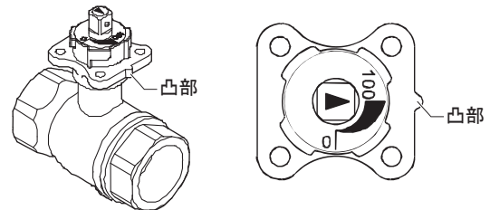
図5 工場出荷時の指針位置
