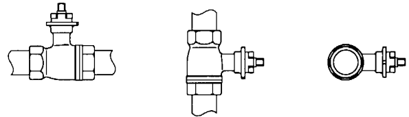
図3 取付姿勢（良い例）
