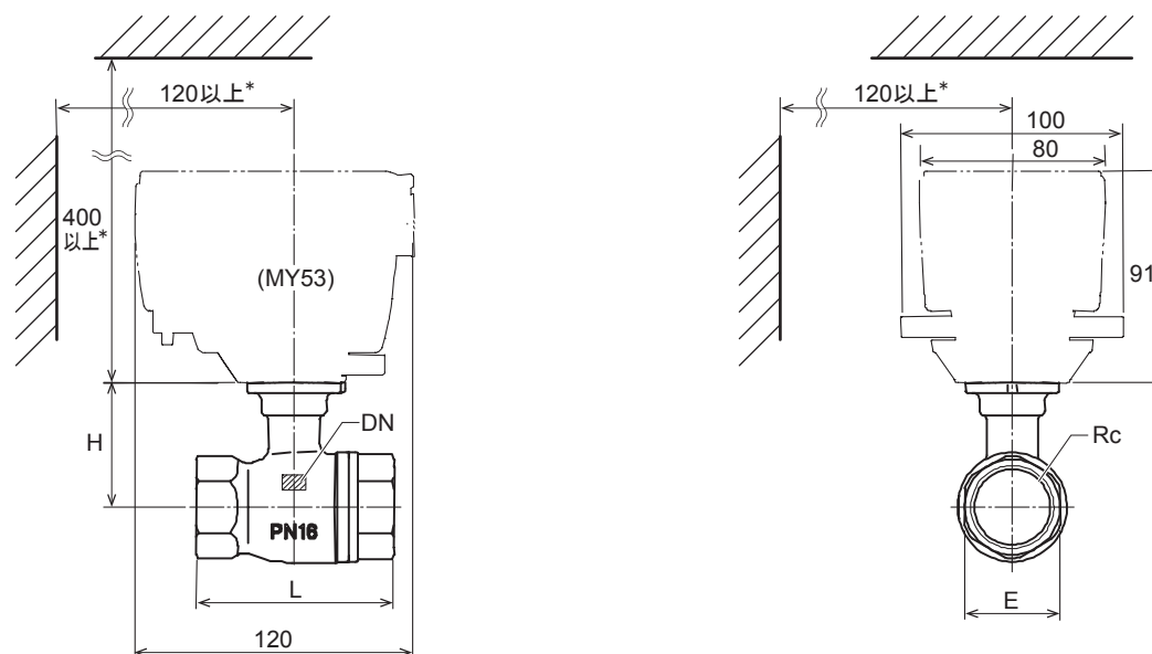
図1 外形寸法図 (mm)
