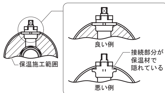
図7 保温施工範囲
