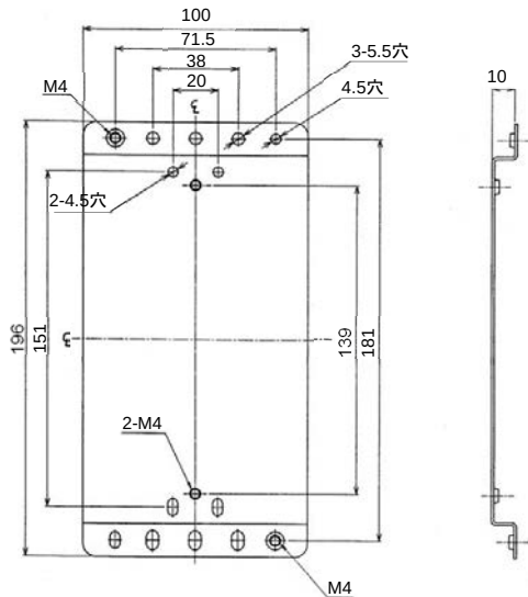
図31 ブラケット小 (形番DY7208A0001) (mm)
