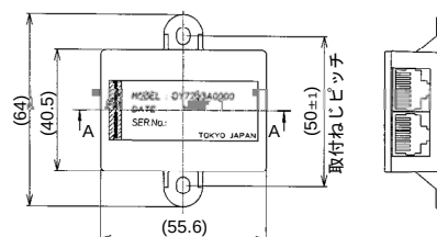
図25 モジュラ分岐ユニット(形番DY7203A0000) (mm)
