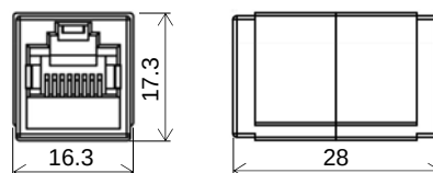
図26 モジュラ中継ユニット(形番DY7202A0000) (mm)
