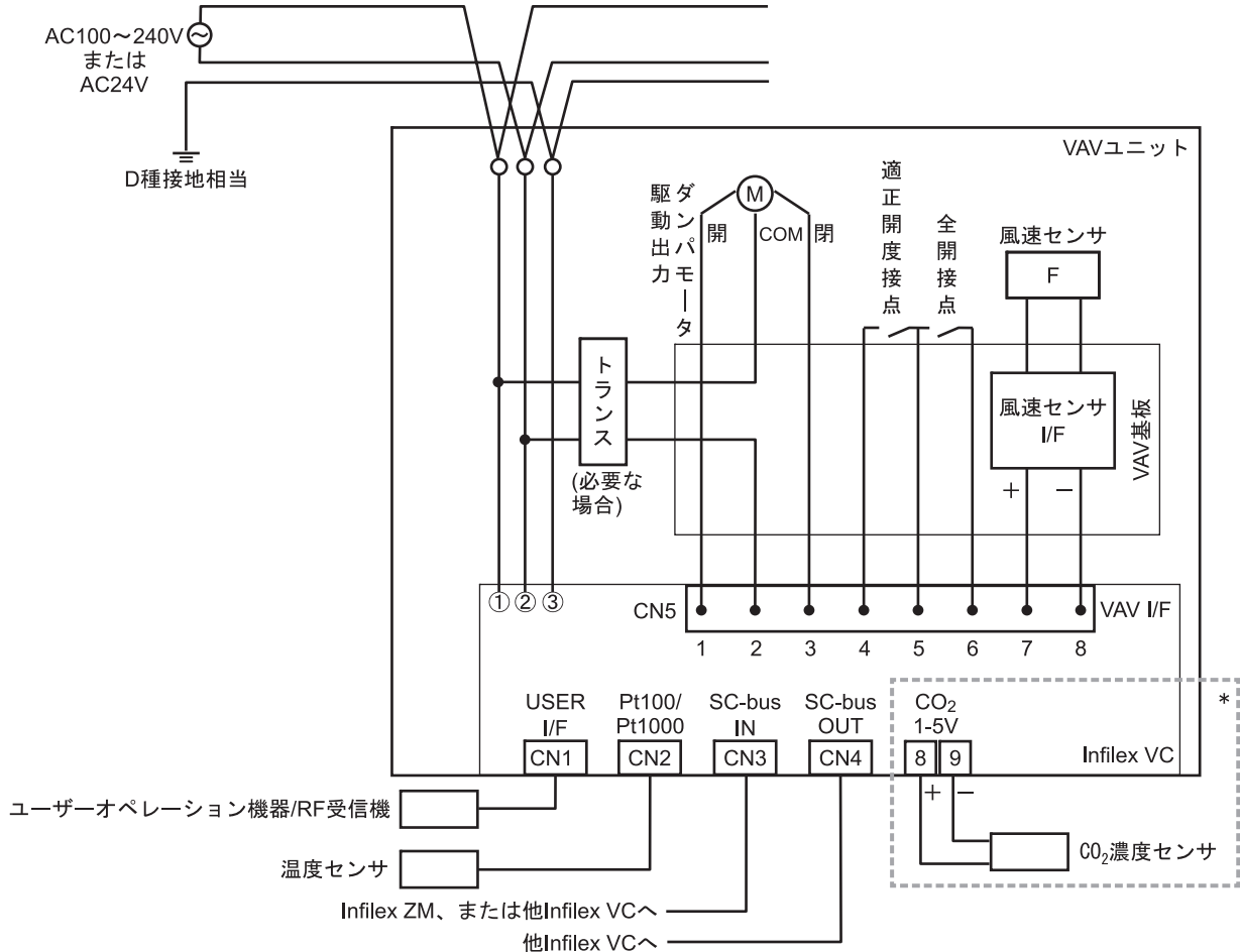
図7 結線図
