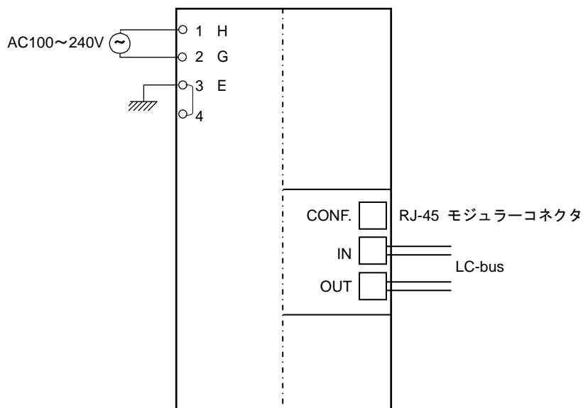
図1 入出力および端子配置図
