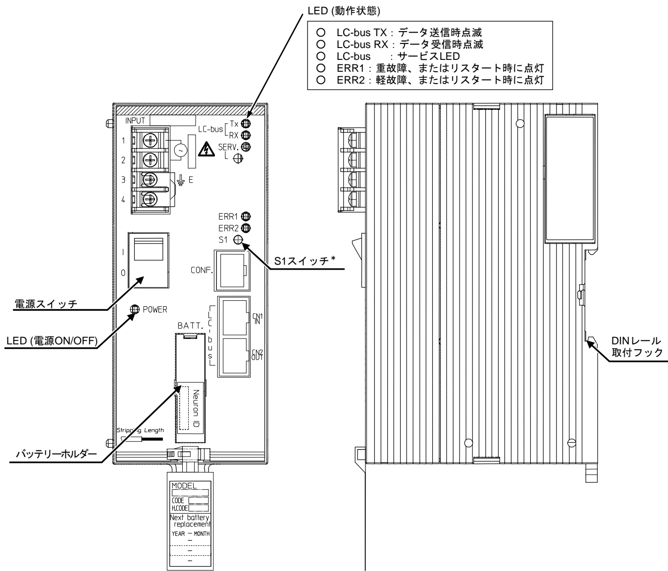
図3 各部の名称
