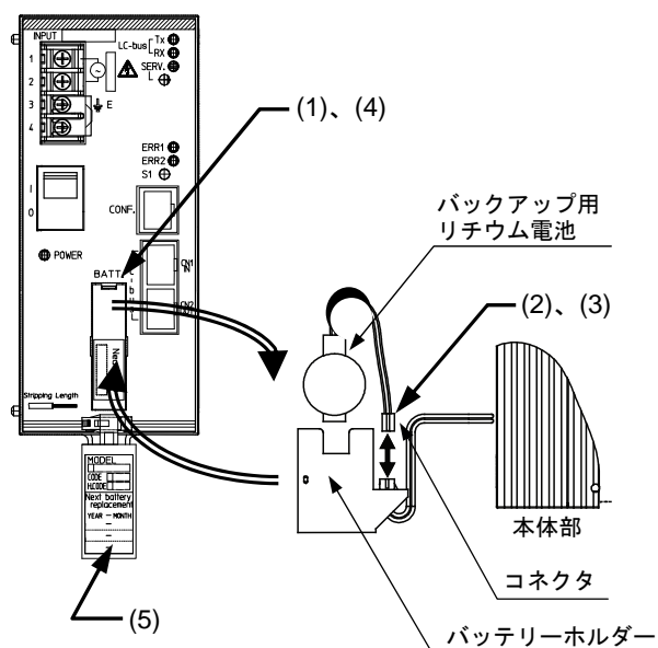
図4 バッテリーの交換方法
