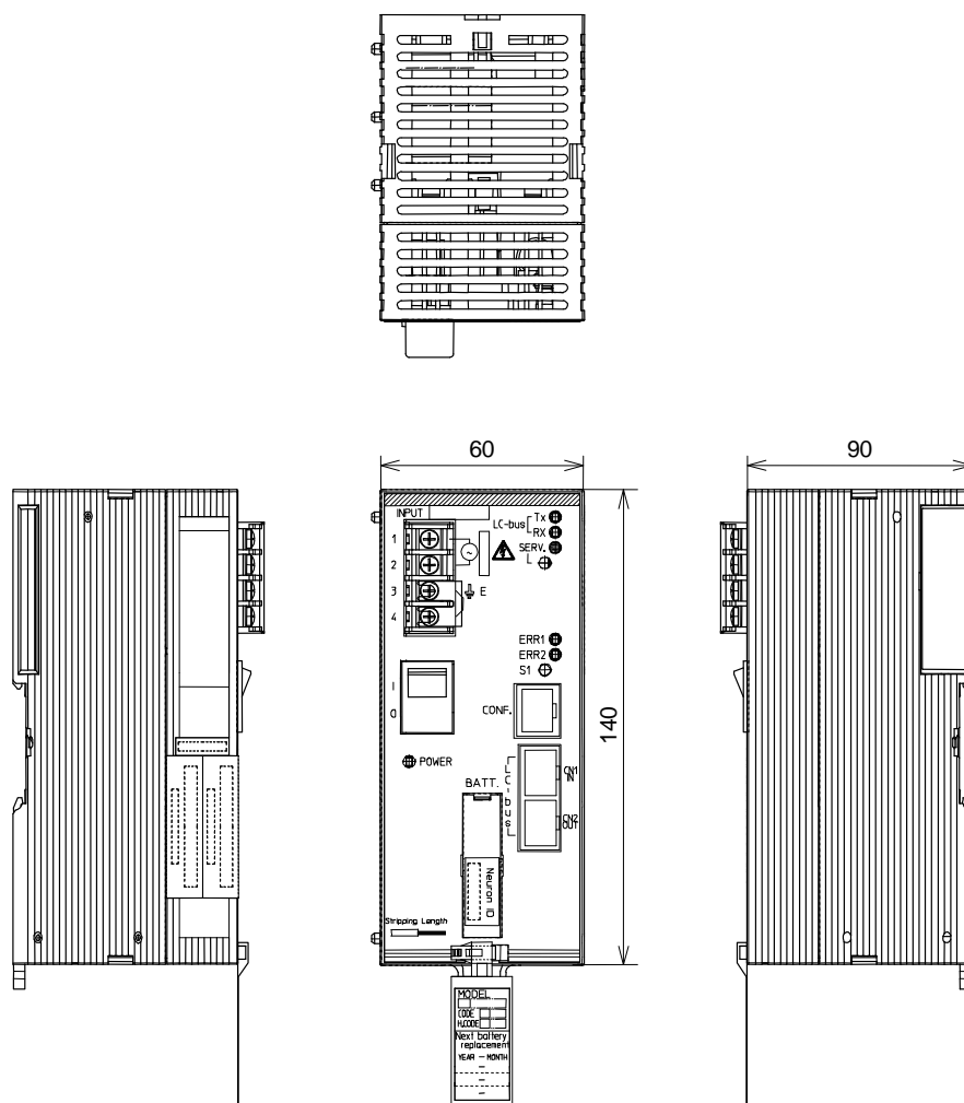
图2 Infilex GC外形寸法图 (mm)
