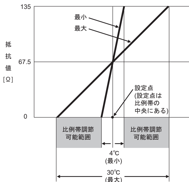
図 10 設定点と比例帯の関係
