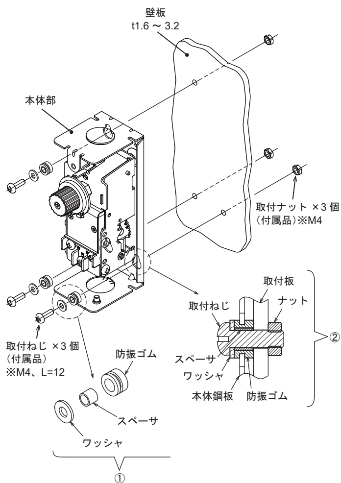
図7 取付手順
