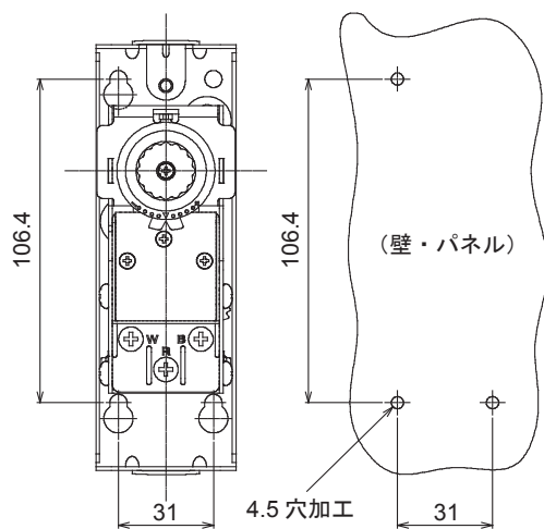
図6 壁板取付寸法 (mm)
