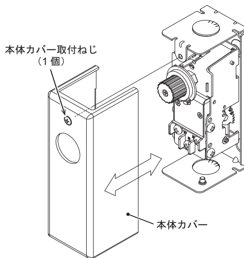
図 5 本体カバーの着脱
