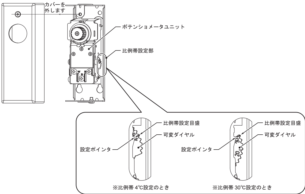
図 11 比例帯調整
