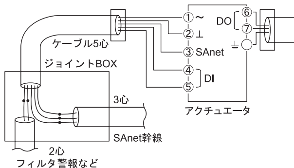
図12 配線の分離
