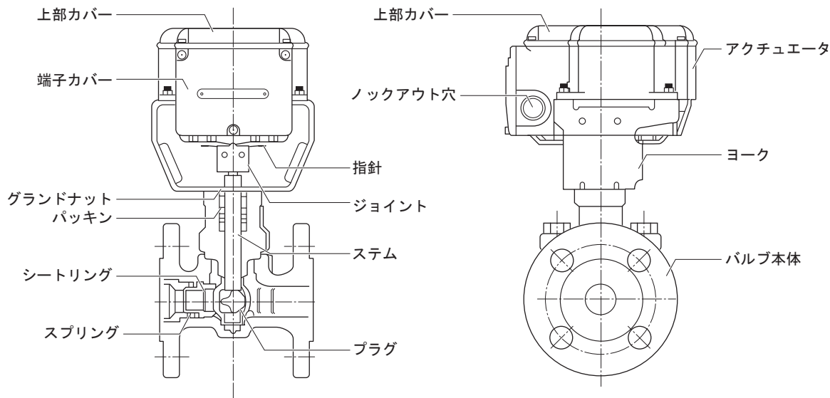
図4 各部の名称
