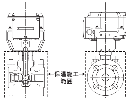
図7 保温施工
