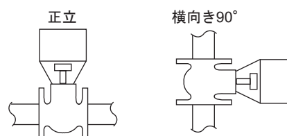
図5 取付姿勢（良い例）
