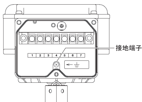
図11 端子台
