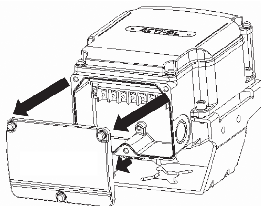
図14 端子カバーの取り外し
