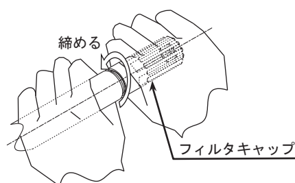
図30 フィルタキャップの取付
