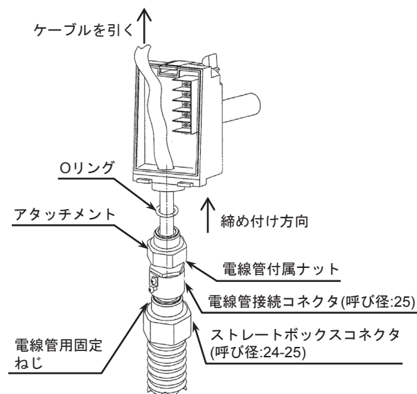
図20 電線管接続
