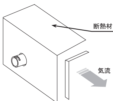
図9 断熱材の施工
