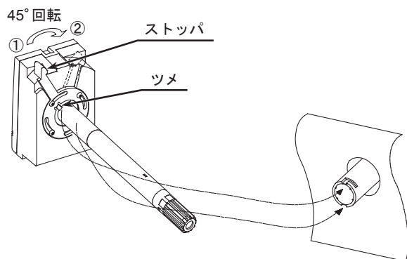
図14 本体の取付
