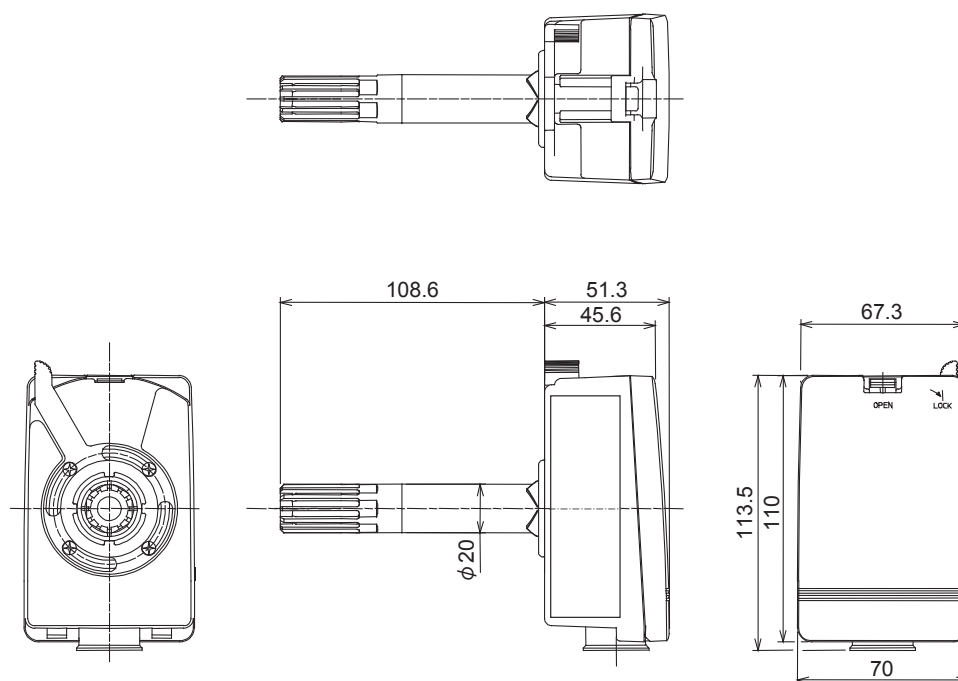
図3 形番H*7813シリーズ (mm)
