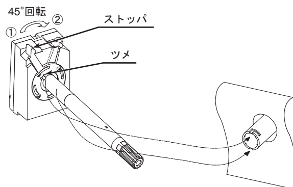
図10 本体の取付
