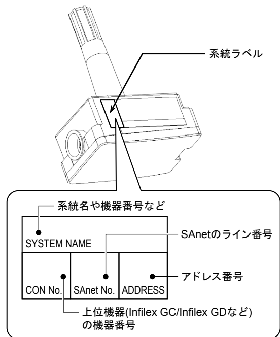
図27 系統ラベル
