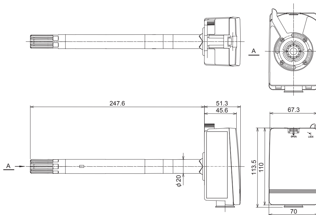
図2 形番H*7803シリーズ (mm)
