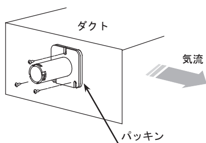
図8 ブラケットの取付
