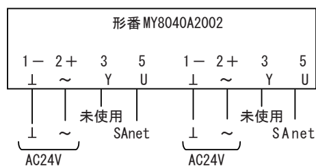
図13 標準タイプ結線図
