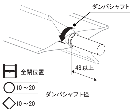
図6 ダンパシャフト
