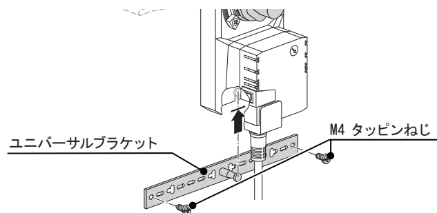
図9 ユニバーサルブラケットの取付
