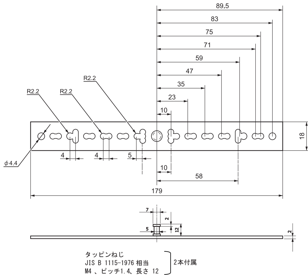
図4 ユニバーサルブラケット (形番12595-00001) 外形寸法図 (mm)
