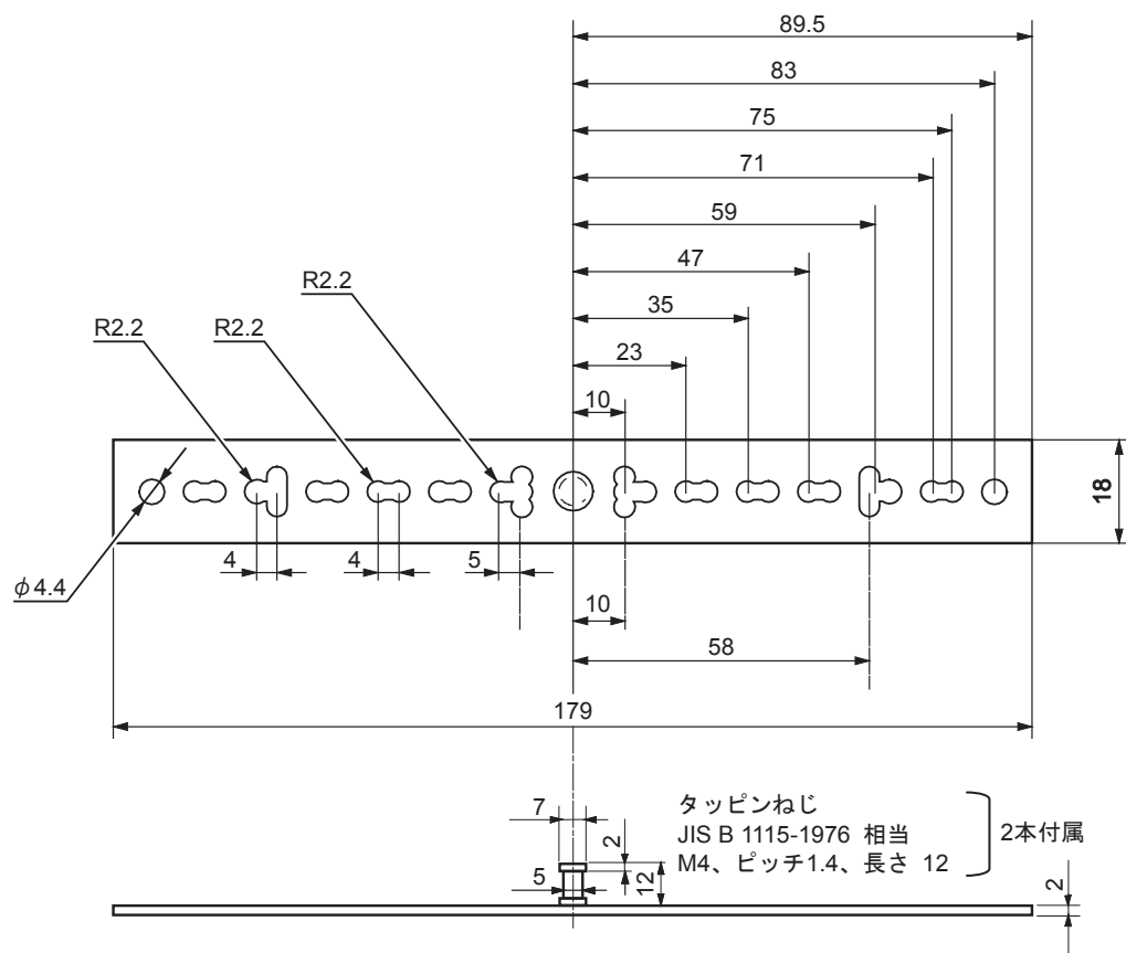
図4 ユニバーサルブラケット (形番12595-00001) 外形寸法図 (mm)
