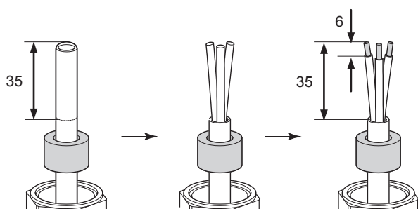
図18 皮膜除去寸法 (mm)
