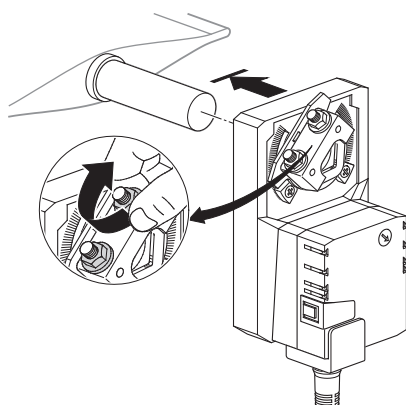
図7 仮止め
