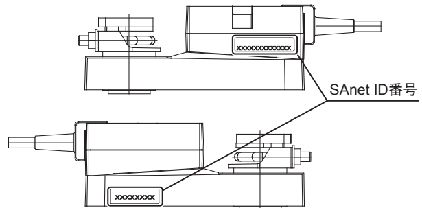
図26 ラベル位置 (標準タイプの場合)
