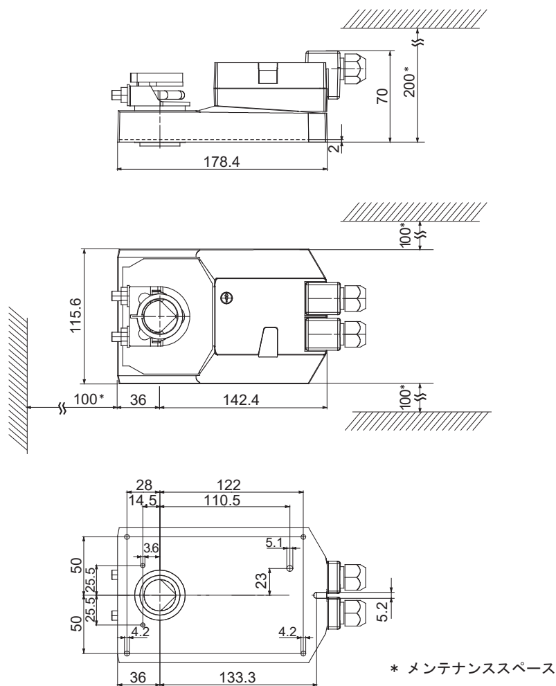
図3 2ターミナルタイプ 外形寸法図 (mm)
