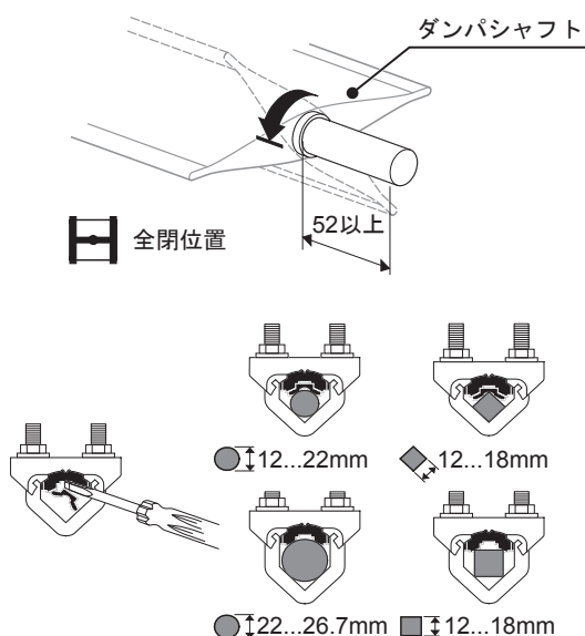
図6 ダンパシャフト
