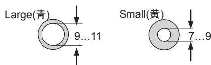
図17 防水コネクタ内部用リング寸法 (mm)
