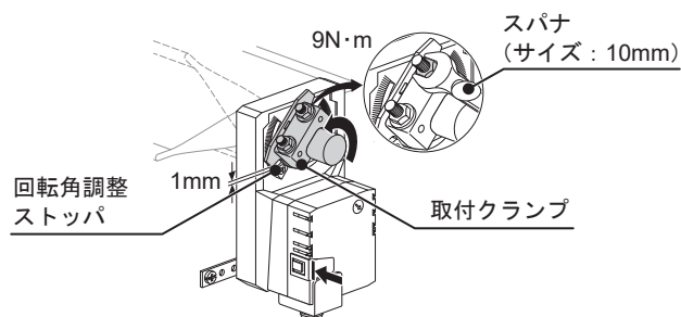
図11 本締め
