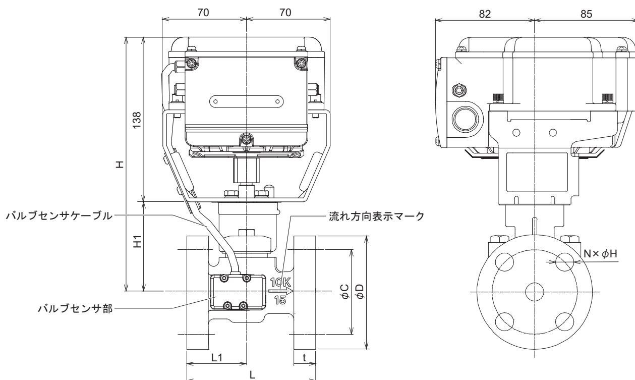
図3 外形寸法図 標準向き（形番FVY5160J00**-B）（単位：mm）
