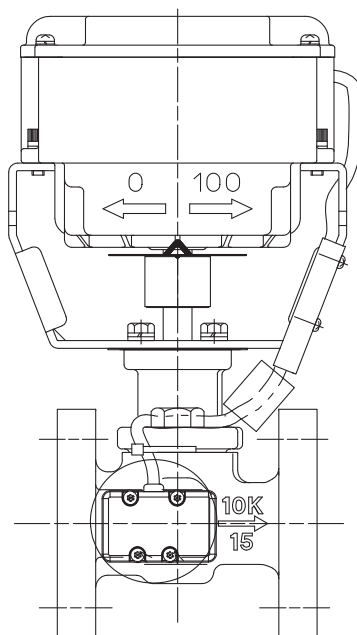
図4 外形図 180°変更 (形番FVY5160J00**-BS1)
