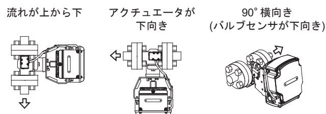
図9 取付姿勢（悪い例）
