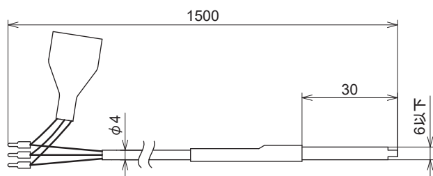
図2 形状・寸法 (mm) モジュラコネクタ出力
