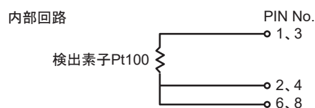
図9 形番TY7820ZMP01内部回路
