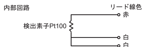
図8 形番TY7820Z0P*内部回路
