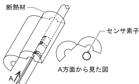
図5 断熱材の取付
