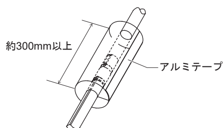
図6 断熱材端面の固定
