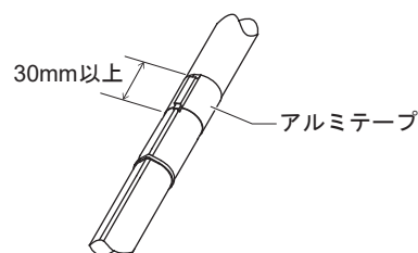
図4 センサ素子部の固定
