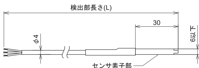
図1 形状・寸法 (mm) リード線出力
