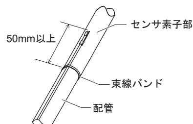
図3 センサの固定
