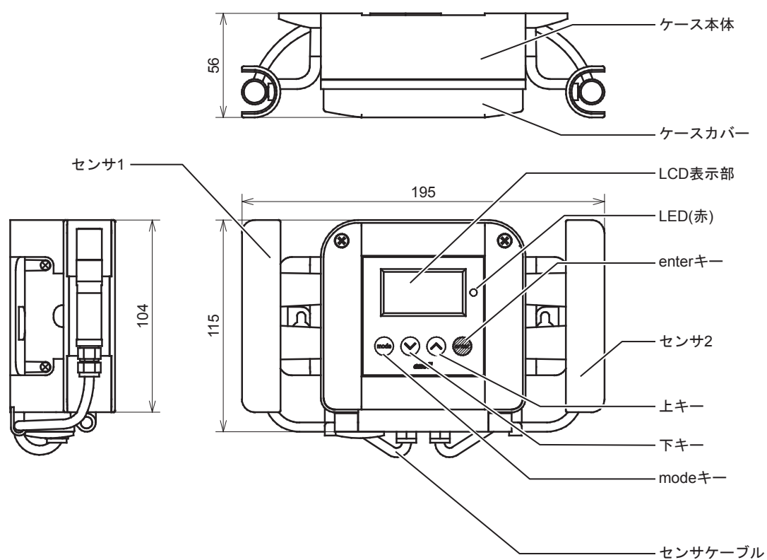
図5 室内取付タイプ 外形寸法図 (mm)
