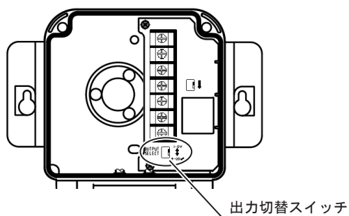
図9 出力切替スイッチ (S1)位置
