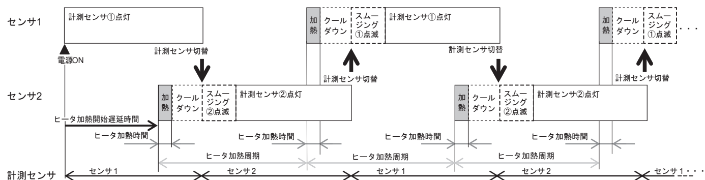
図29 電源ON後の基本動作 (センサ1が計測センサで始まった場合)
