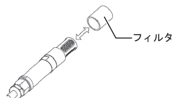
図34 フィルタ交換
