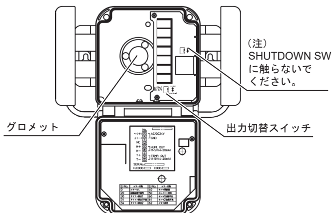
図14 グロメット位置
