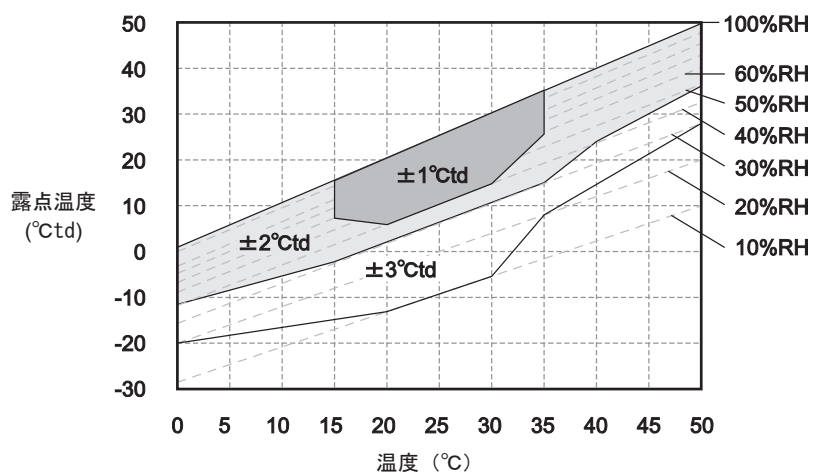
図3 室内用 露点温度精度
