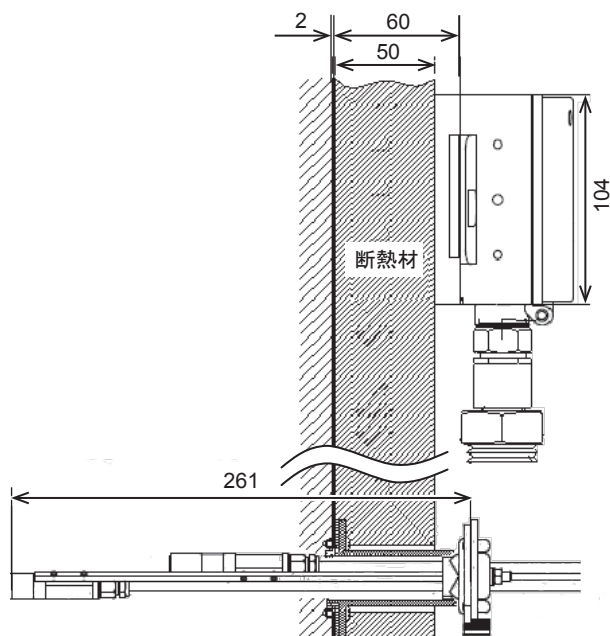
図23 ダクト用 取付詳細図
