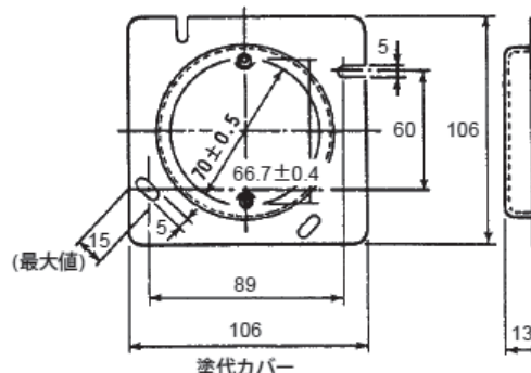
JIS規格塗代付きカバー外形寸法 (mm) (中形四角ボックス用・市販品)
