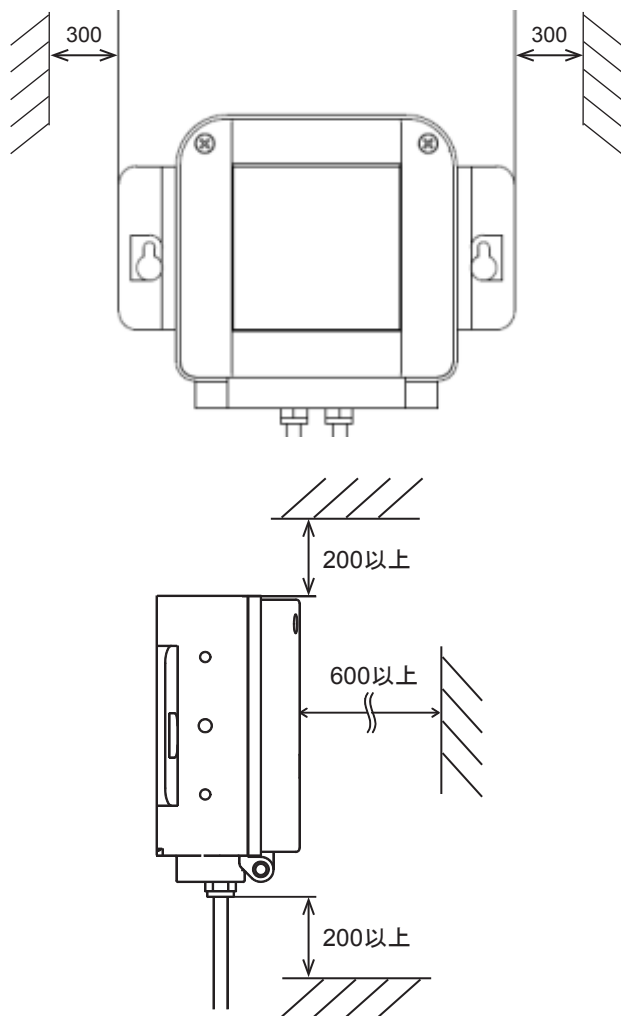
図12 メンテナンススペース
