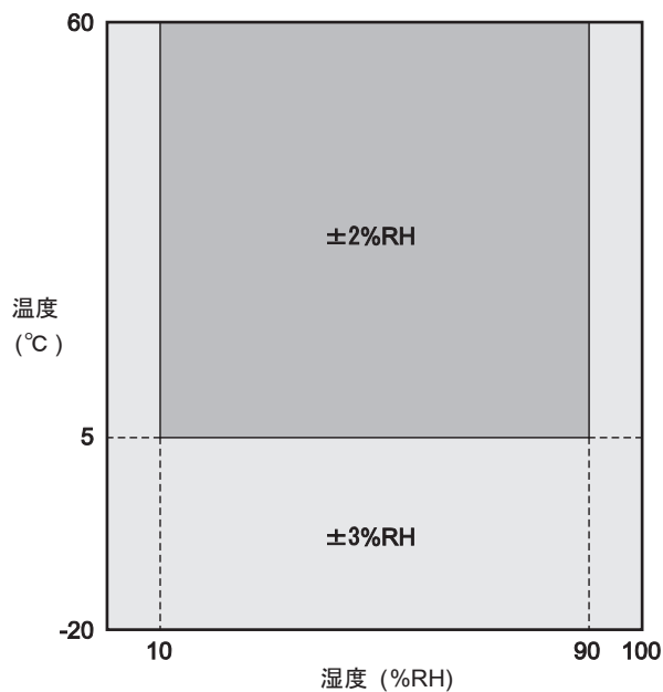
図2 ダクト用 湿度精度
