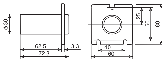
図7 ダクト用取付ブラケット 外形寸法図 (mm)
