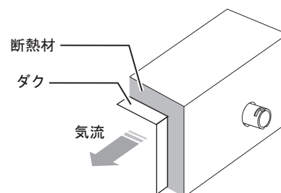
図19 断熱材の施工
