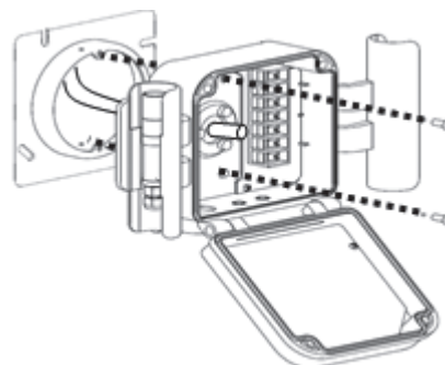
図15 ケースの取付
