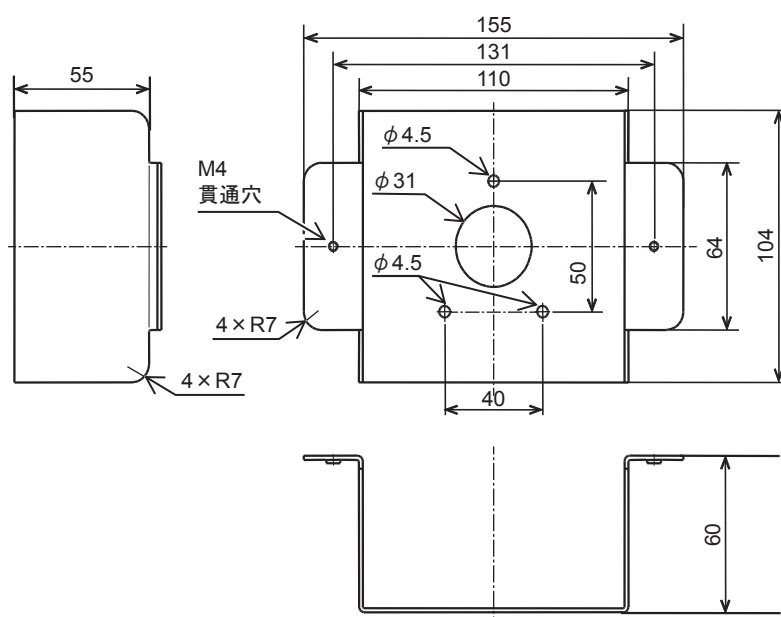
図8 ダクト用本体取付ブラケット 外形寸法図 (mm)
