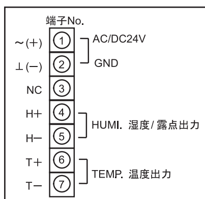
図27 結線図
