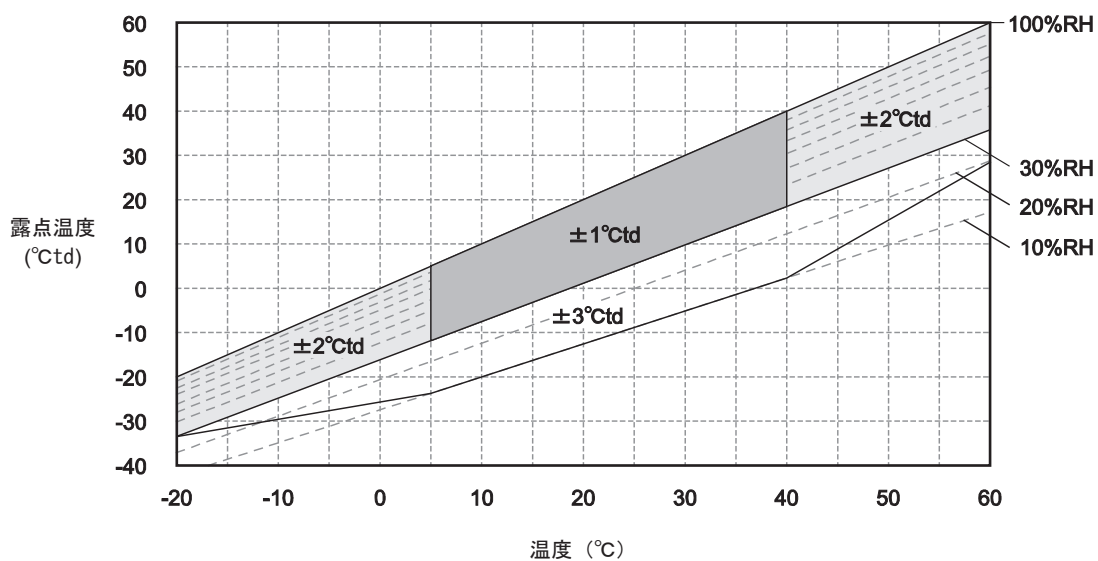
図4 ダクト用 露点温度精度 (ケース周囲温度25°C)
