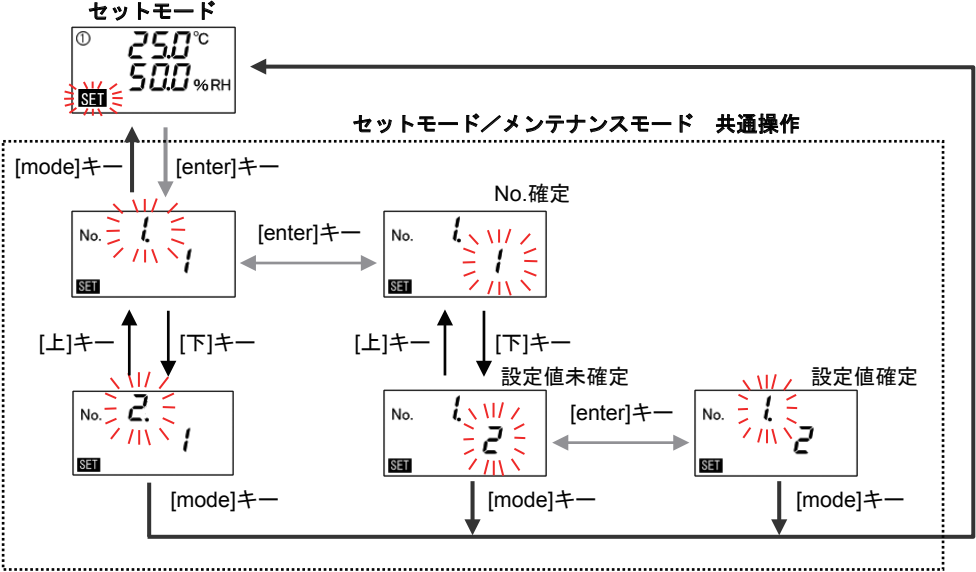
図31 操作モード関連図 (セットモードの場合)
