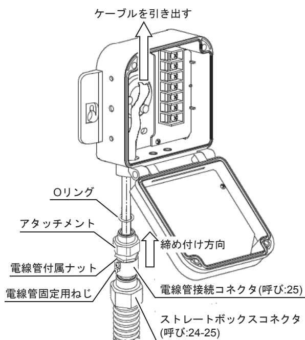
図25 電線管取付
