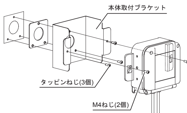
図20 ケースの取り付け
