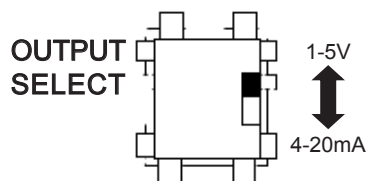
図10 出力切替スイッチ (S1)
