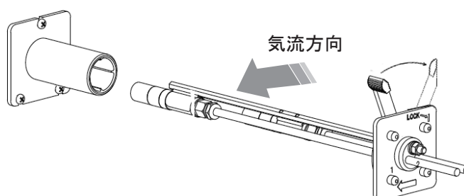
図11 気流方向
