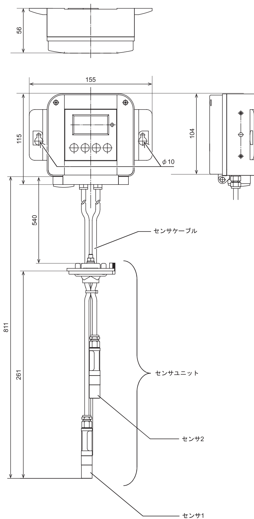
図6 ダクト取付タイプ 外形寸法図 (mm)
