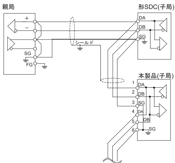
図25 RS-485用 5線式
