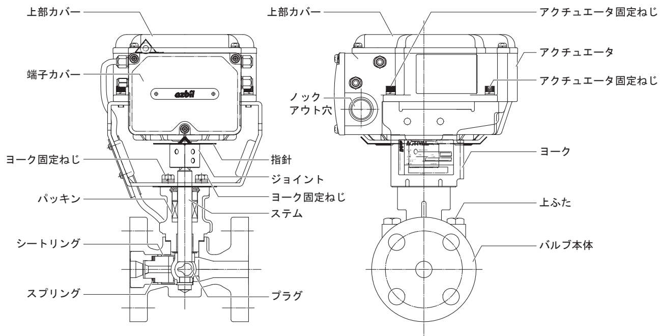
図4 各部の名称
