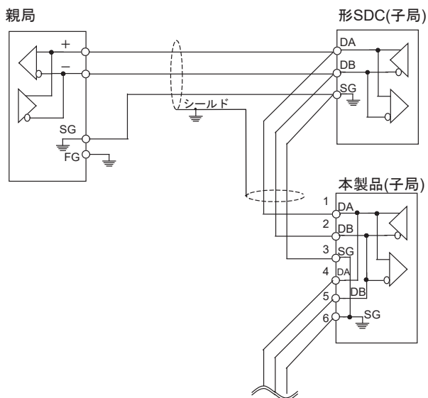
図24 RS-485用 3線式
