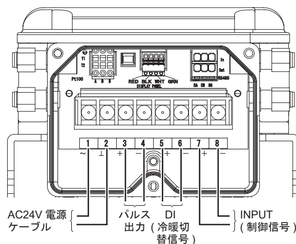
図12 基本配線接続
