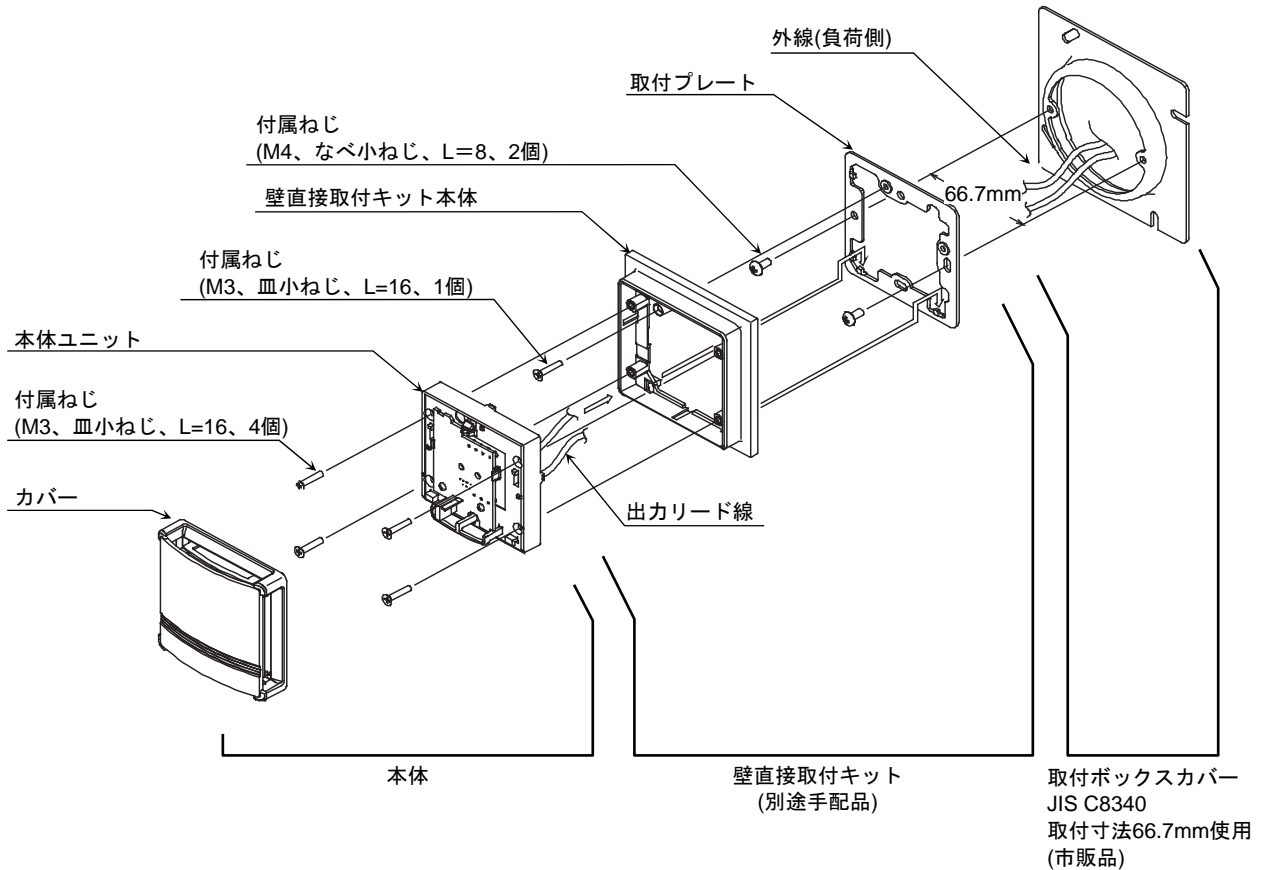
図5 取付手順 壁直接取付キットによる取付
