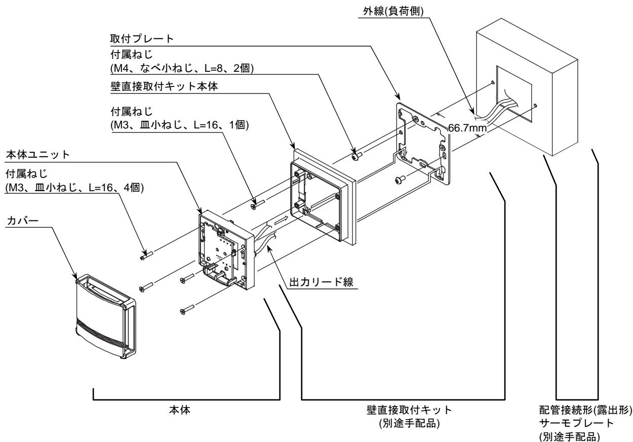
図6 取付手順 配管接続形サーモプレート取付
