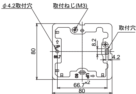
図2 取付プレート寸法表面図 (mm)
