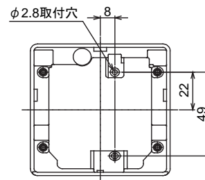
図4 サーモプレート取付キットの取付表面寸法図 (mm)
