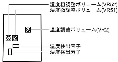
図16 調整ボリュームの基板上的位置 (形TY7043D、形HY7043D、形HTY7043D)
