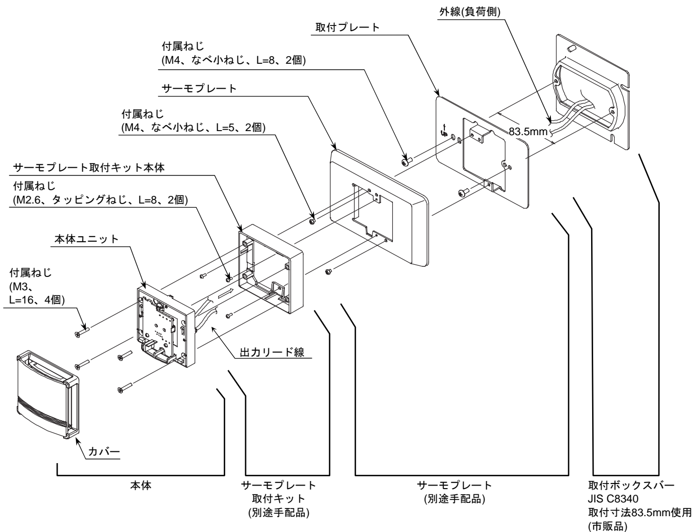
図8 取付手順 サーモプレート取付キットによる取付
