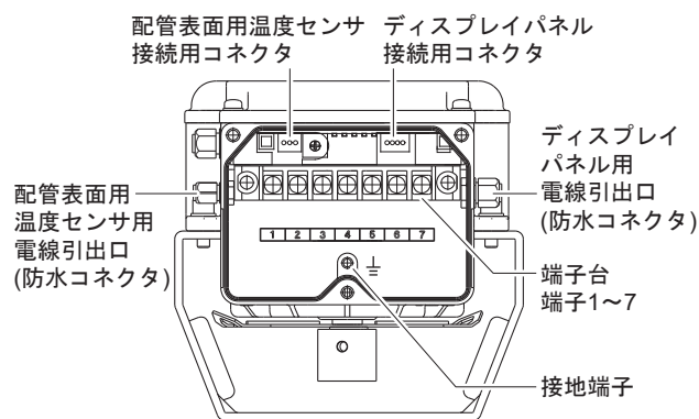
図16 接続部と端子台
