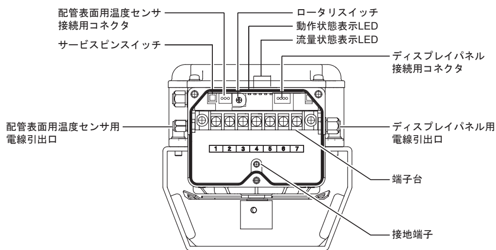
図7 接続部・表示部詳細
