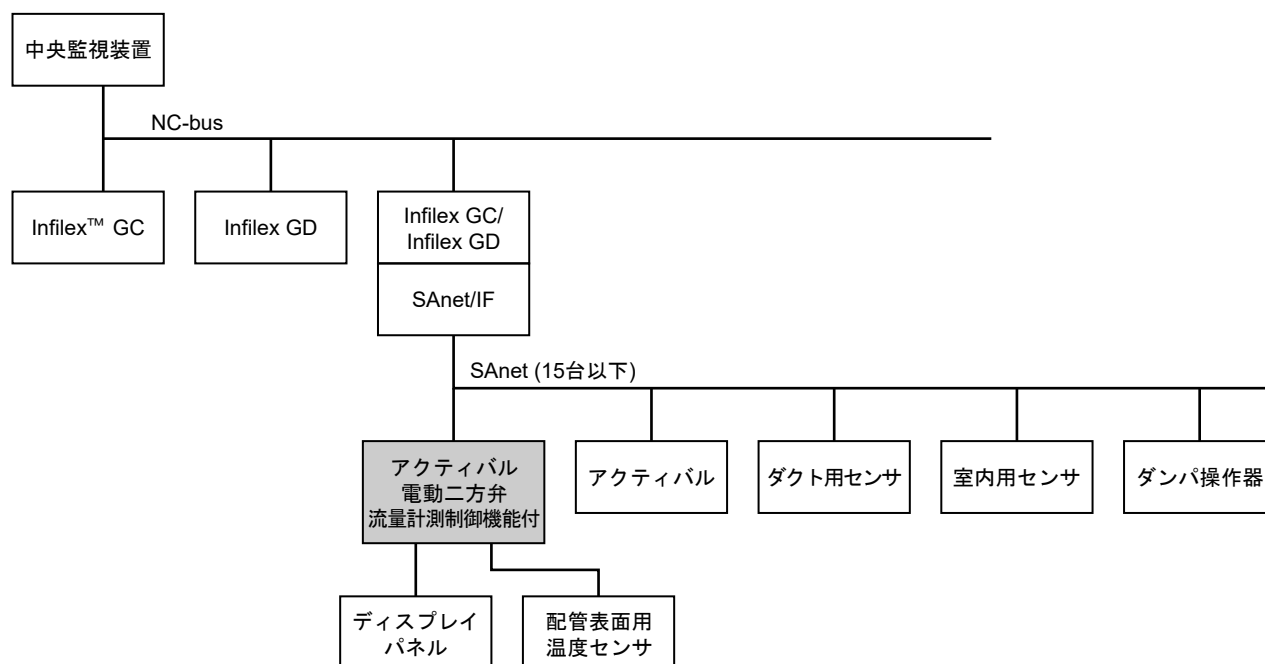
図2 システム構成例：savic-net FX2
