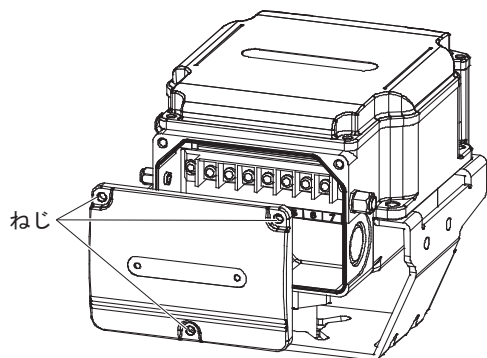
図20 端子カバーの取り外し
