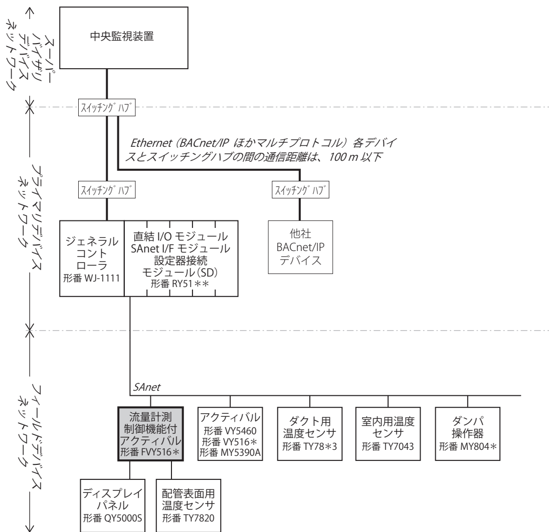
図1 システム構成例：savic-net G5
