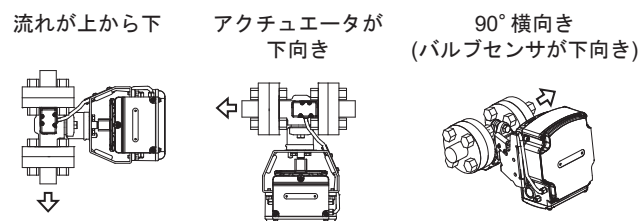
図9 取付姿勢（悪い例）
