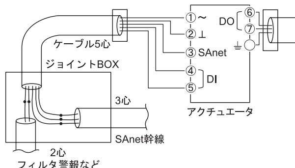
図17 配線の分離
