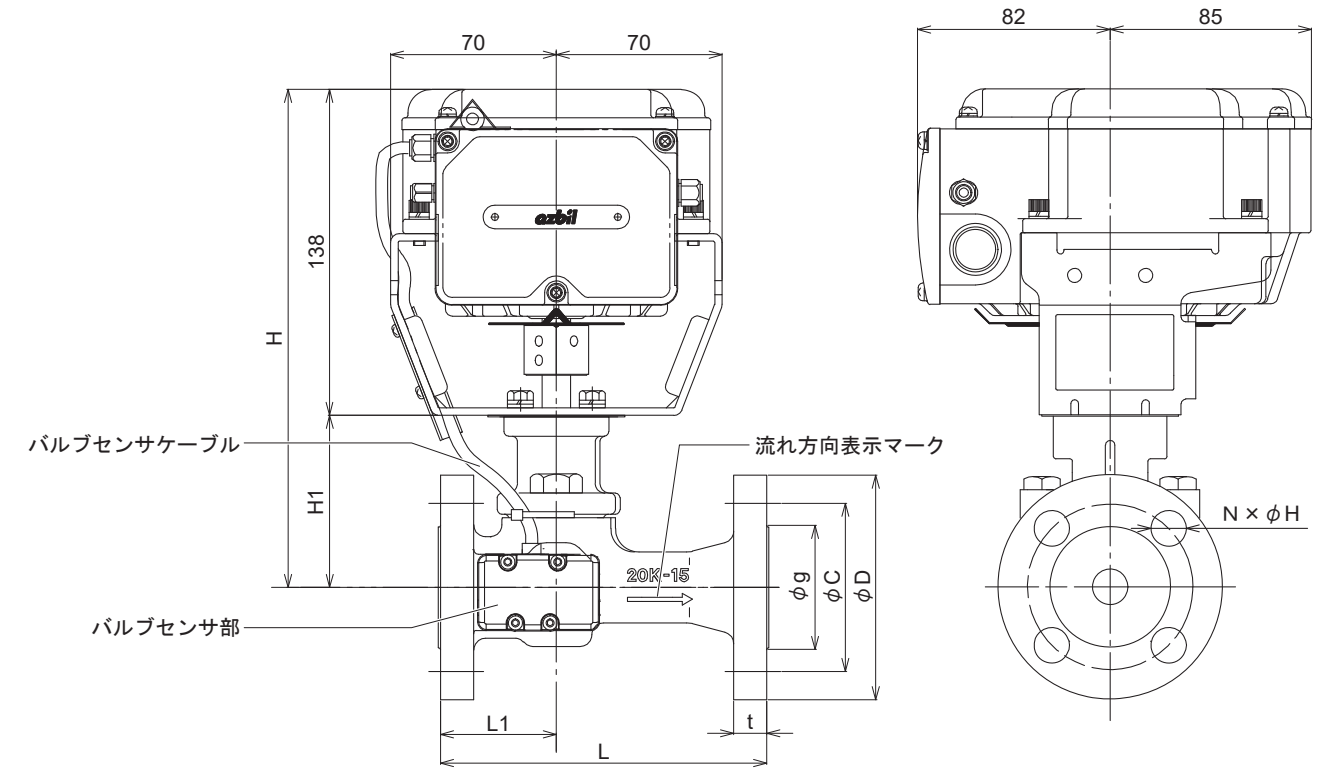
図3 外形寸法図 標準向き（形番FVY516EJ00**-B）（単位：mm）
