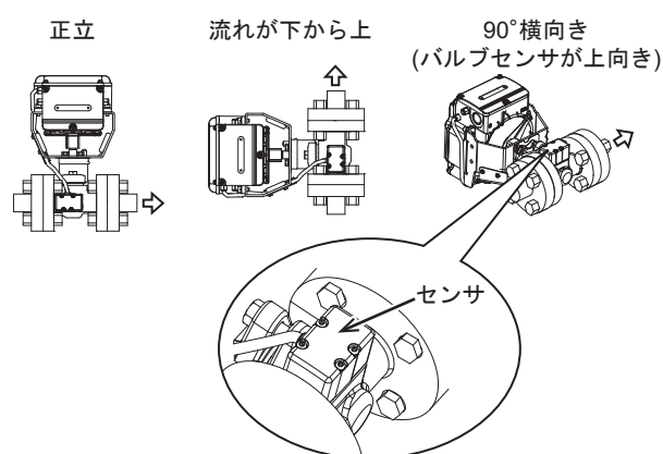
図8 取付姿勢（良い例）
