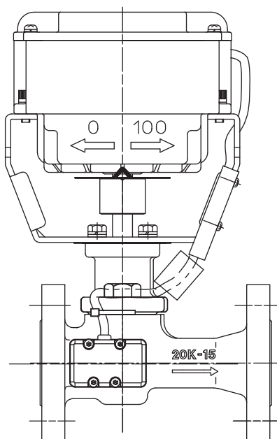
図4 外形図 180° 変更 (形番FVY516EJ00**-BS1)
