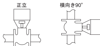
図 3 取付姿勢（良い例）
