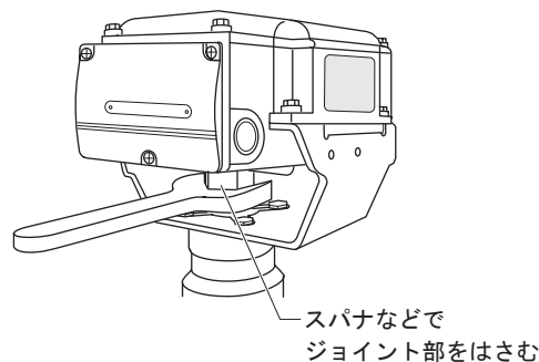
図7 手動開閉操作
