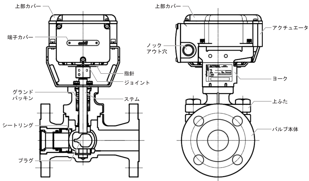
図2 各部の名称
