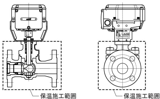
図5 保温施工
