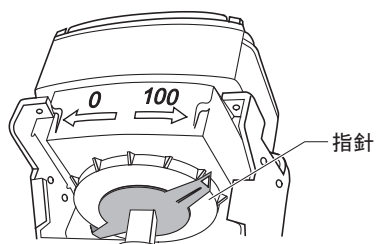
図6 工場出荷時の指針位置
